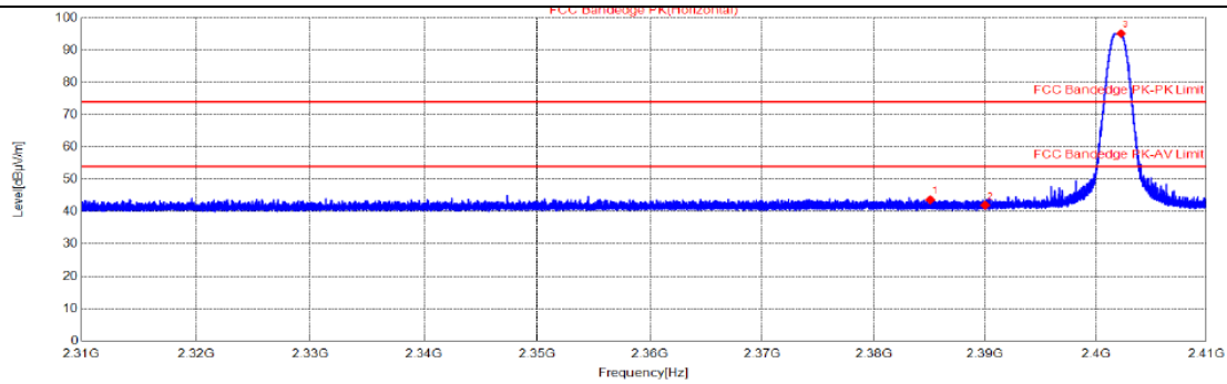
BLE_2402_Ant1/ Horizontal
