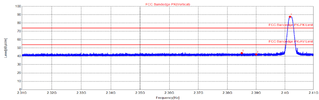
BLE_2402_Ant1/ Vertical
