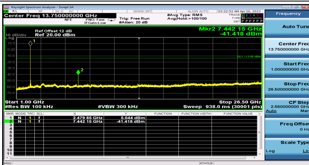
ZIGB_Ant1_2480_1000~26500
