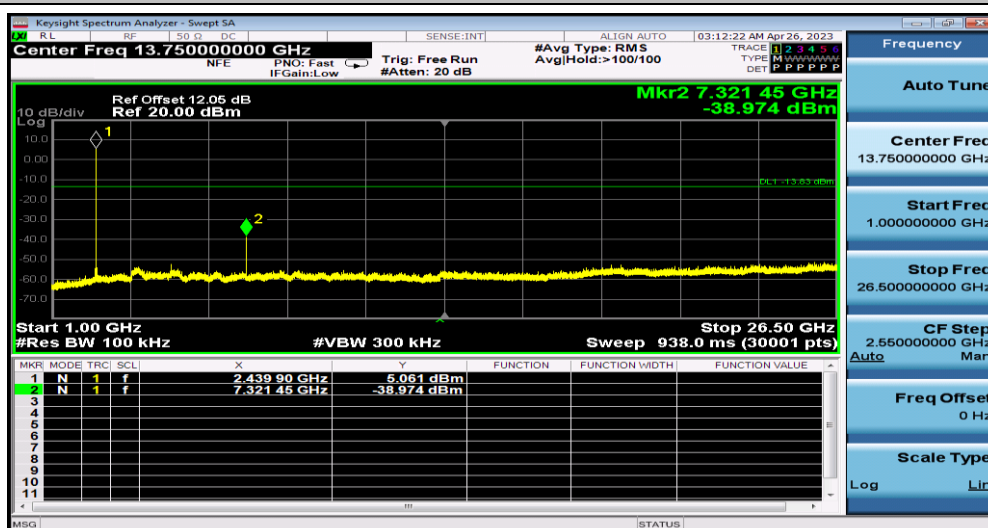
ZIGB_Ant1_2440_1000~26500
