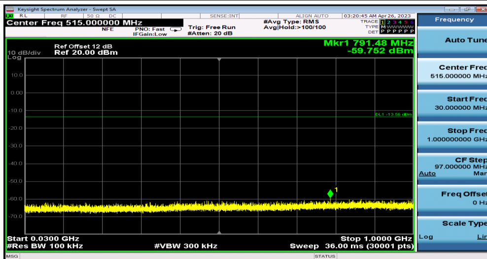
ZIGB_Ant1_2480_30~1000
