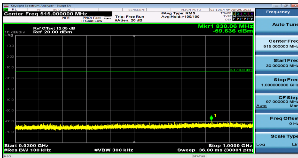
ZIGB_Ant1_2440_30~1000
