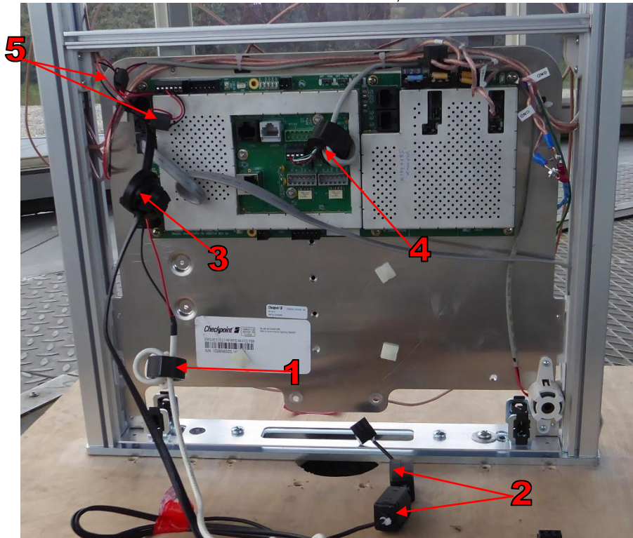
Evolve E10 2.0 ANT RF, Submaster
