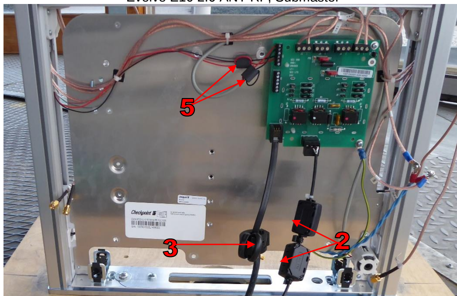
Evolve E10 2.0 ANT RF, Submaster
