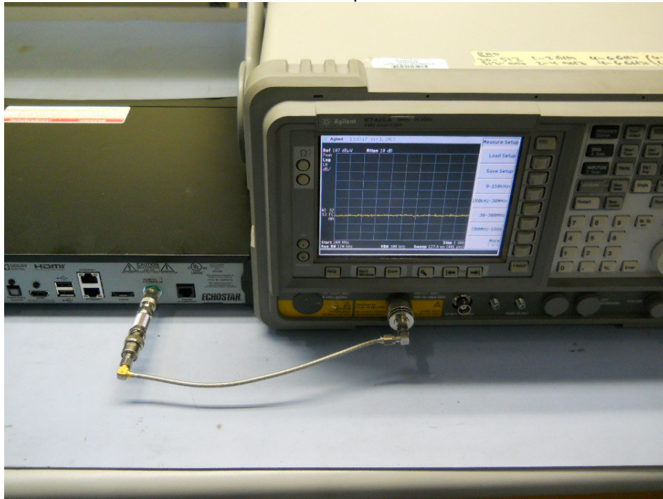
RF4CE port
