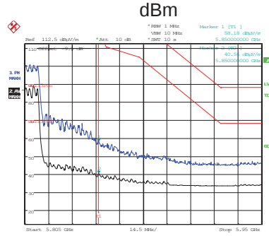
Channel 159 BW=40MHz MCS9NSS1 48q
