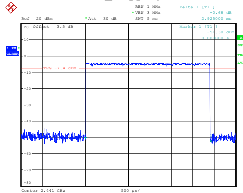
2DH5_Hopping 2.925ms
