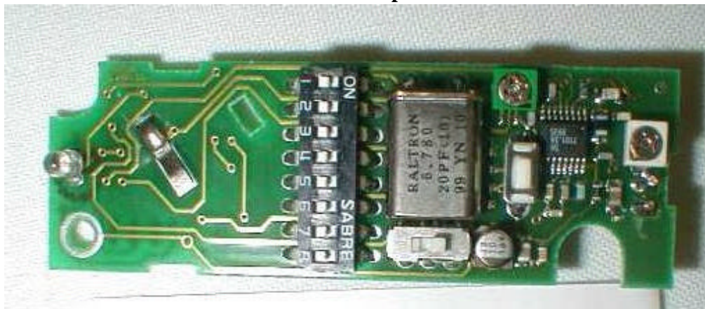
PCB Top
