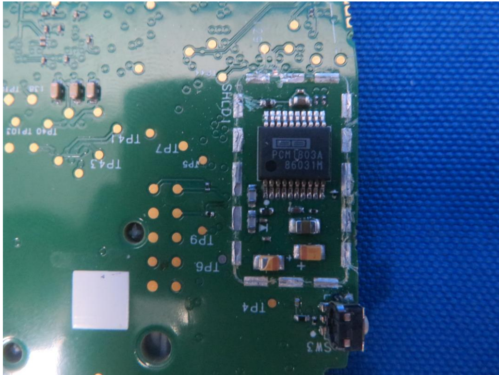
(10) EUT Photo (SLXD1 G58)
