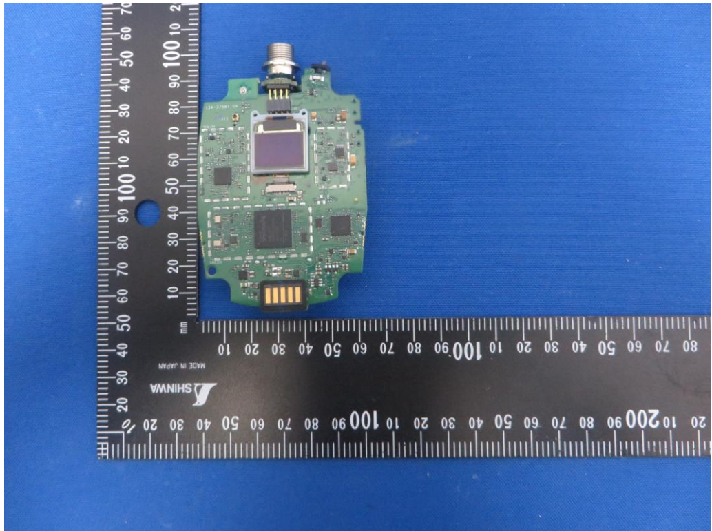
(4) EUT Photo (SLXD1 G58)
