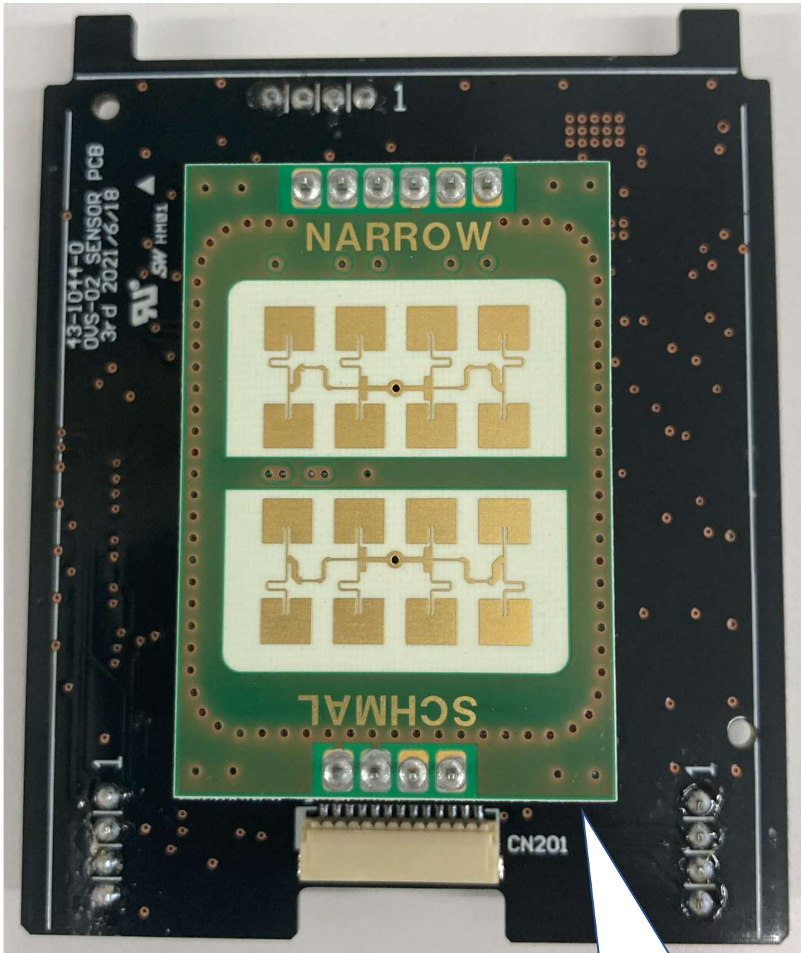
RADIO MODULE
