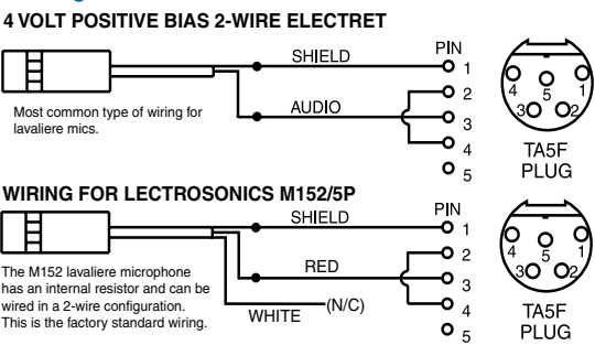
Fig. 3 - DPA Microphones
