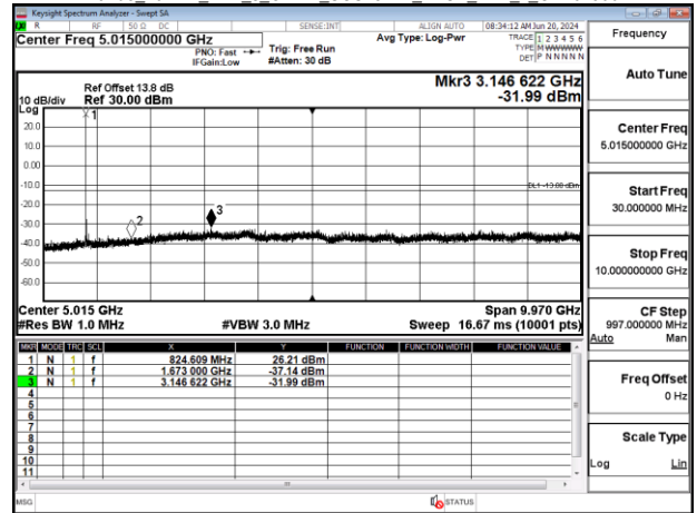
Band5 10MHz DFT s_OFDM_SCS15kHz_BPSK_RB1_1_CH168800
