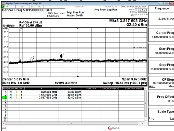
Band5 15MHz DFT s OFDM_SCS15kHz_BPSK_RB1_1_CH168300
