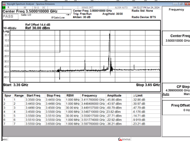
Band77-Part27_100MHz_CP_OFDM_SCS30kHz_QPSK_RB1_272_CH633334
