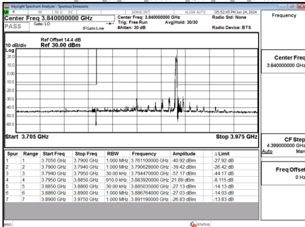
Band77-Part27_90MHz_CP_OFDM_SCS30kHz_QPSK_RB1_244_CH656000
