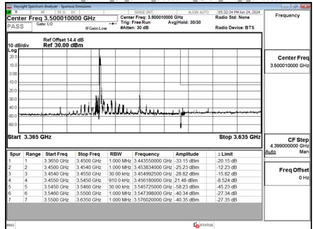
Band77-Part27_90MHz_CP_OFDM_SCS30kHz_QPSK_RB1_0_CH633334
