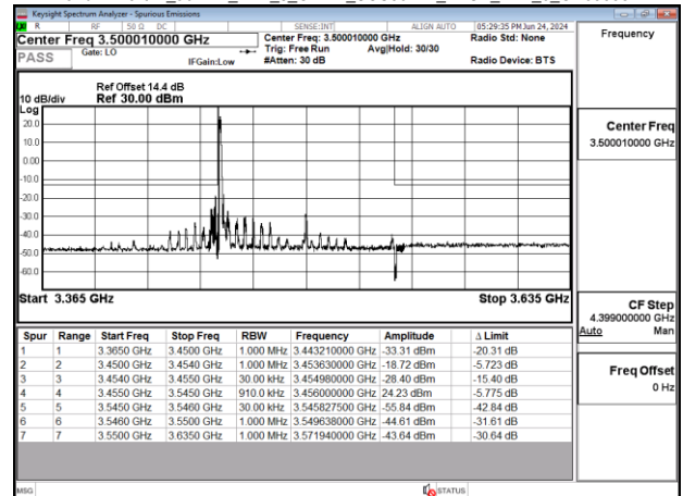
Band77-Part27_90MHz_DFT_s_OFDM_SCS30kHz_BPSK_RB1_0_CH633334
