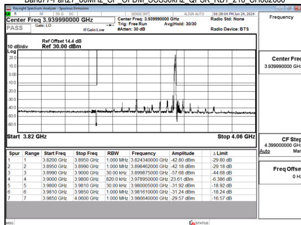
Band77-Part27_80MHz_CP_OFDM_SCS30kHz_QPSK_RB217_0_CH632668
