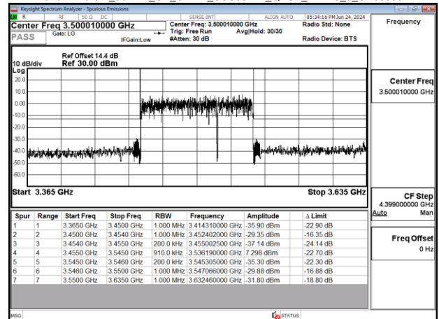
Band77-Part27_90MHz_CP_OFDM_SCS30kHz_QPSK_RB245_0_CH633334
