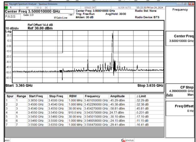
Band77-Part27_90MHz_CP_OFDM_SCS30kHz_QPSK_RB1_244_CH633334
