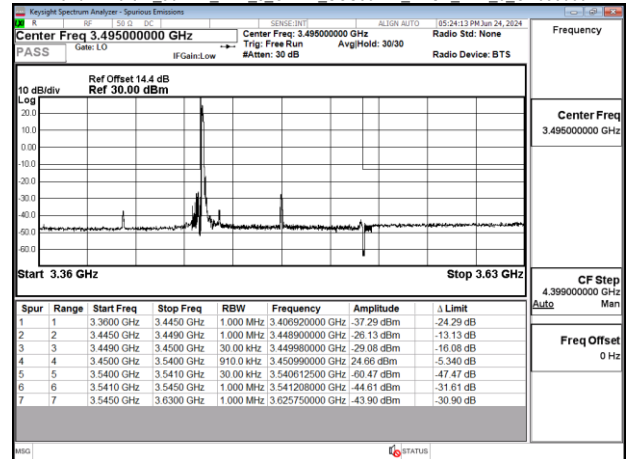
Band77-Part27_90MHz_DFT_s_OFDM_SCS30kHz_BPSK_RB1_0_CH633334
