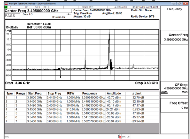
Band77-Part27_90MHz_CP_OFDM_SCS30kHz_QPSK_RB1_244_CH633334
