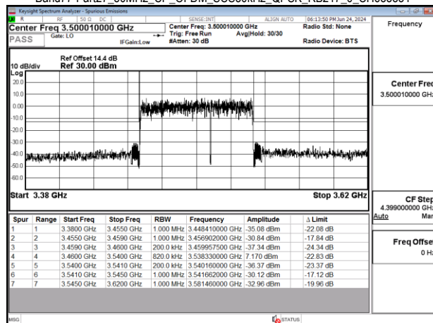
Band77-Part27_80MHz_CP_OFDM_SCS30kHz_QPSK_RB217_0_CH633334
