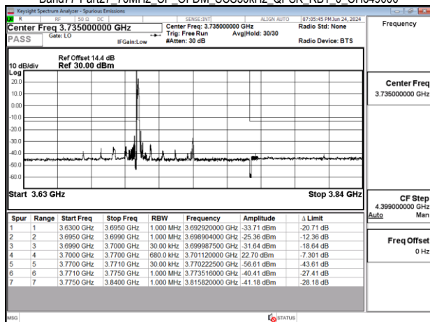
Band77-Part27_70MHz_CP_OFDM_SCS30kHz_QPSK_RB1_0_CH656000
