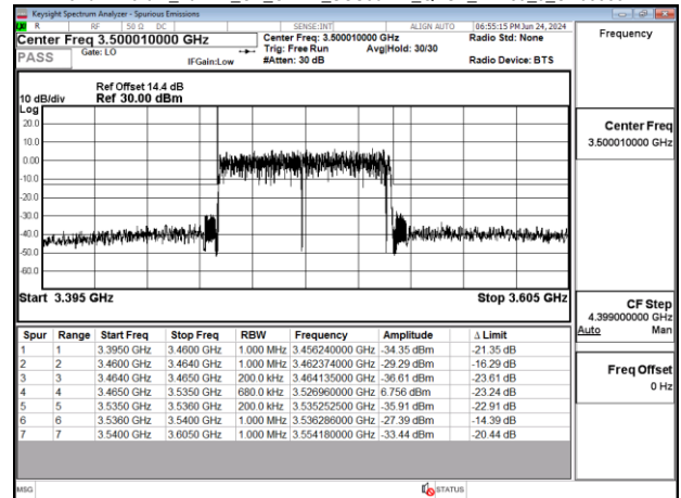
Band77-Part27_70MHz_CP_OFDM_SCS30kHz_QPSK_RB189_0_CH633334
