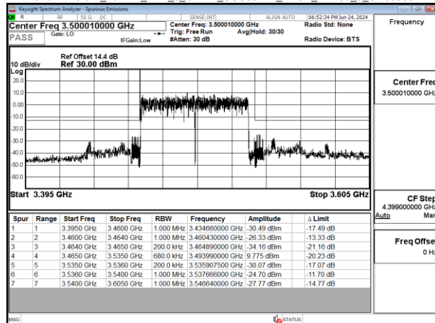
Band77-Part27_70MHz_DFT_s_OFDM_SCS30kHz_BPSK_RB180_0_CH633334
