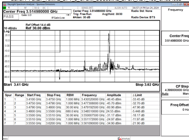
Band77-Part27_70MHz_DFT_s_OFDM_SCS30kHz_BPSK_RB1_188_CH649000
