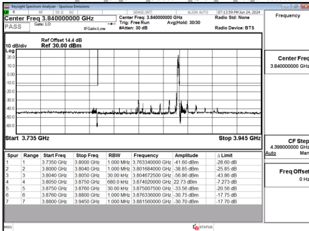
Band77-Part27_70MHz_CP_OFDM_SCS30kHz_QPSK_RB1_188_CH656000
