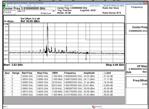
Band77-Part27_80MHz_CP_OFDM_SCS30kHz_QPSK_RB1_216_CH632668
