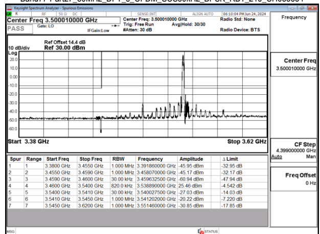
Band77-Part27_80MHz_DFT_s_OFDM_SCS30kHz_BPSK_RB1_216_CH633334
