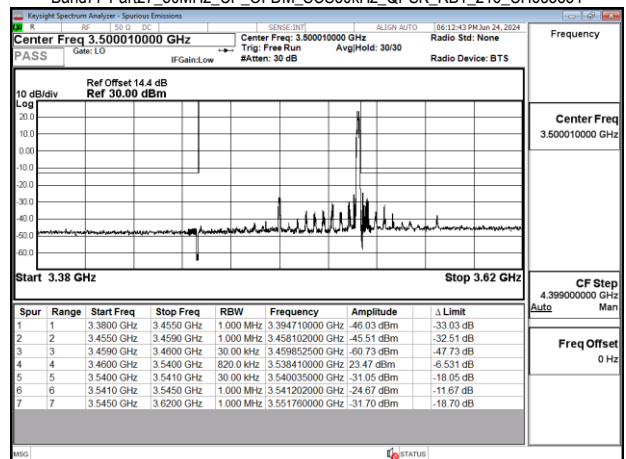
Band77-Part27_80MHz_CP_OFDM_SCS30kHz_QPSK_RB1_216_CH633334
