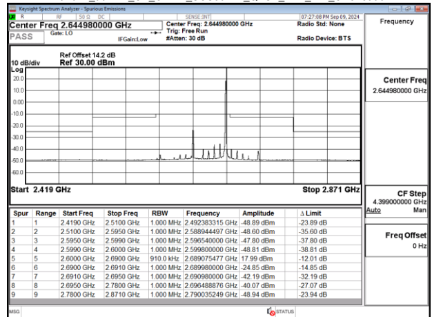
Band41_90MHz_CP_OFDM_SCS30kHz_QPSK_RB1_244_CH528996
