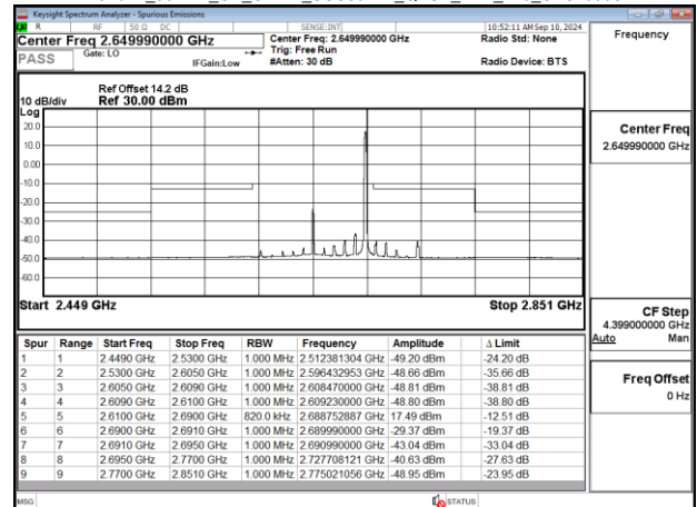
Band41 80MHz CP OFDM_SCS30kHz QPSK RB1_216_CH529998
