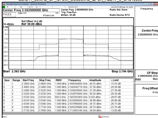
Band41 80MHz CP OFDM SCS30kHz QPSK RB217 0 CH518598
