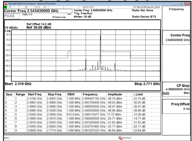
Band41_90MHz_CP_OFDM_SCS30kHz_QPSK_RB1_244_CH518598
