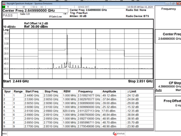
Band41 80MHz CP OFDM_SCS30kHz QPSK RB1_216_CH507204
