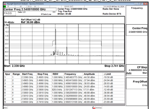
Band41 80MHz CP OFDM SCS30kHz QPSK RB1 0 CH508002
