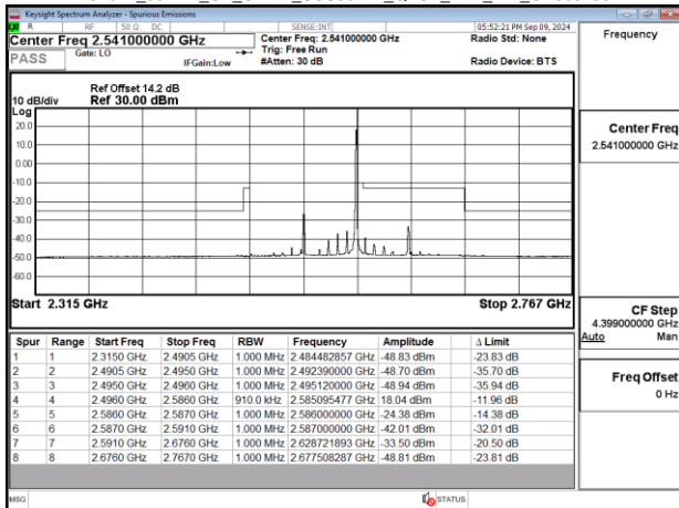
Band41_90MHz_CP_OFDM_SCS30kHz_QPSK_RB1_244_CH508200
