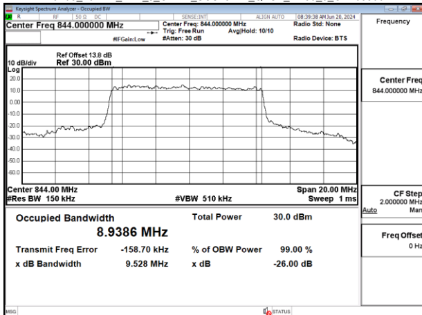
Band5_10MHz_DFT_s_OFDM_SCS15kHz_QPSK_RB50_0_CH168800
