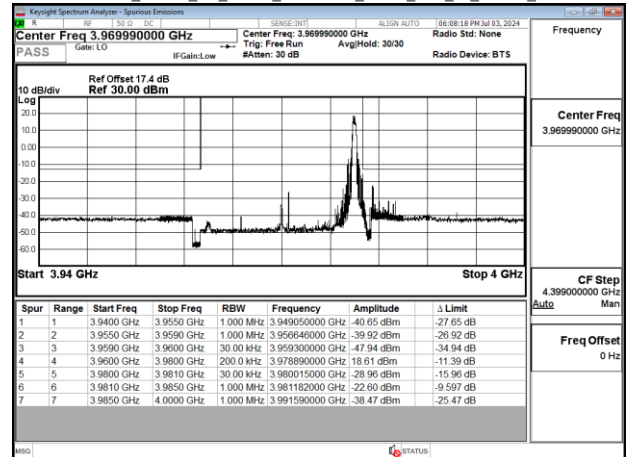
Band77-Part27_20MHz_CP_OFDM_SCS30kHz_QPSK_RB1_50_Chain0_CH664666
