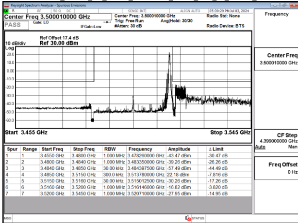
Band77-Part27_30MHz CP OFDM_SCS30kHz QPSK RB1_77_Chain0_CH635666
