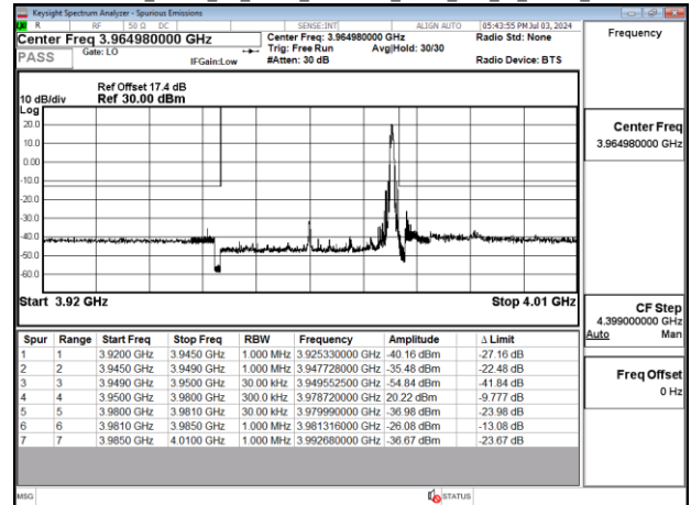
Band77-Part27_30MHz CP OFDM_SCS30kHz QPSK RB1_77_Chain0_CH664332
