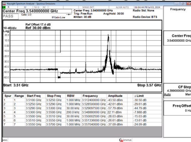
Band77-Part27_20MHz_CP_OFDM_SCS30kHz_QPSK_RB1_50_Chain0_CH636000
