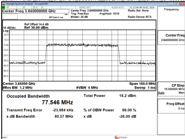
Band77-Part27 80MHz CP OFDM SCS30kHz 256QAM RB217_0 Chain1_CH656000
