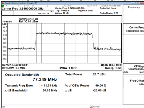
Band77-Part27 80MHz CP OFDM SCS30kHz 16QAM RB217_0 Chain1 CH656000
