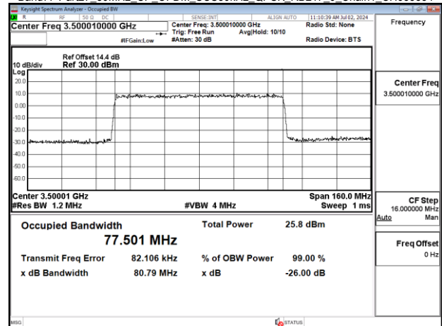
Band77-Part27_80MHz_CP_OFDM_SCS30kHz_QPSK_RB217_0_Chain1_CH633334
