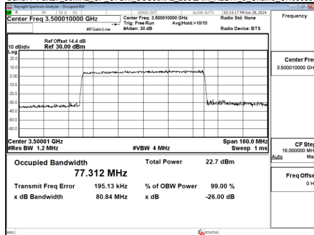
Band77-Part27 80MHz CP OFDM SCS30kHz 256QAM RB217_0 Chain0_CH633334
