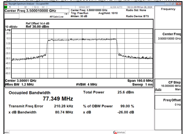
Band77-Part27 80MHz CP OFDM SCS30kHz 64QAM RB217_0 Chain0 CH633334
