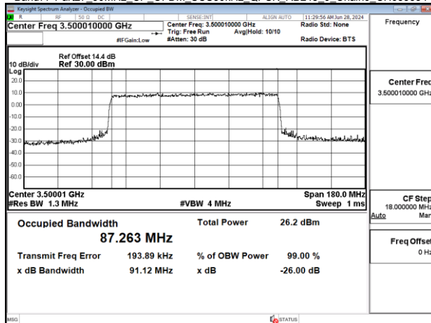
Band77-Part27 90MHz CP OFDM SCS30kHz QPSK RB245_0 Chain0_CH633334
