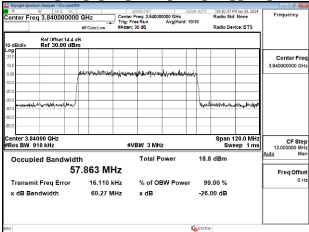
Band77-Part27 60MHz CP OFDM SCS30kHz 256QAM RB162_0 Chain0_CH656000
