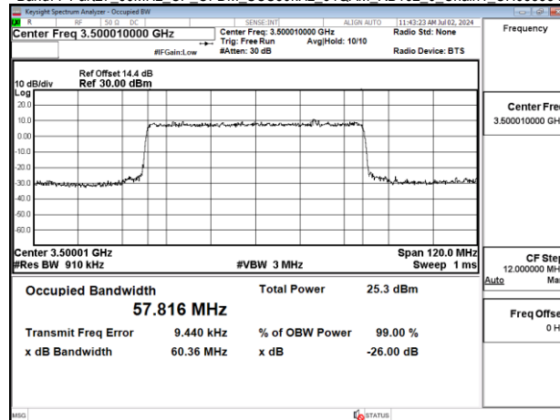
Band77-Part27 60MHz CP OFDM SCS30kHz 64QAM RB162_0 Chain1_CH633334
