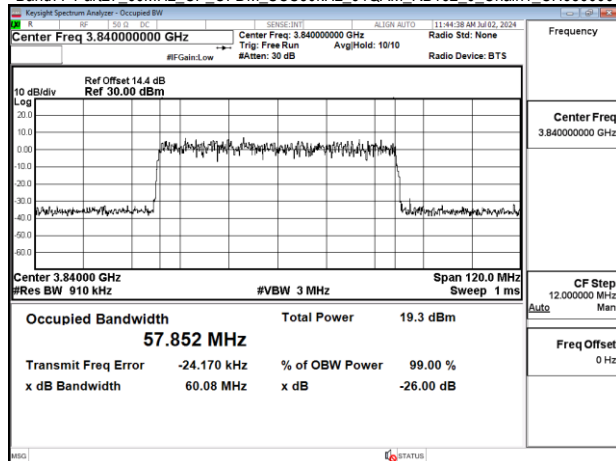
Band77-Part27 60MHz CP OFDM SCS30kHz 64QAM RB162_0 Chain1_CH656000
