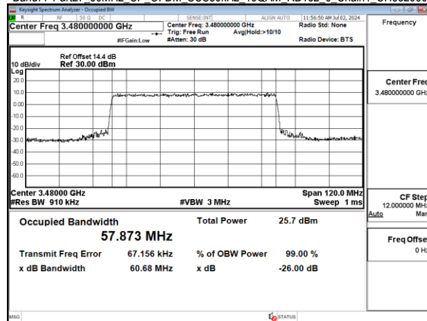
Band77-Part27 60MHz CP OFDM SCS30kHz 16QAM RB162_0 Chain1_CH633334
