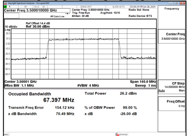
Band77-Part27 70MHz CP OFDM SCS30kHz QPSK RB189_0 Chain0 CH633334
