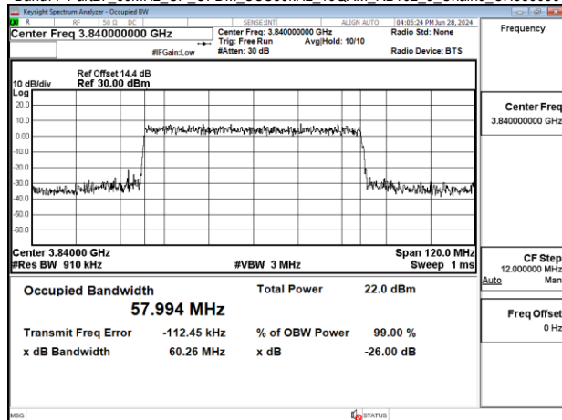
Band77-Part27 60MHz CP OFDM SCS30kHz 16QAM RB162_0 Chain0_CH656000
