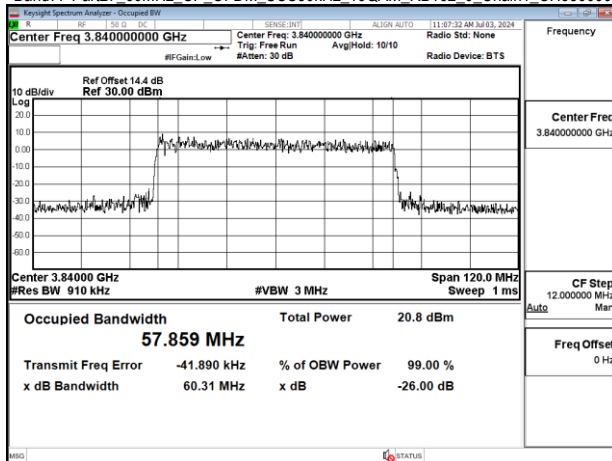
Band77-Part27 60MHz CP OFDM SCS30kHz 16QAM RB162_0 Chain1_CH656000
