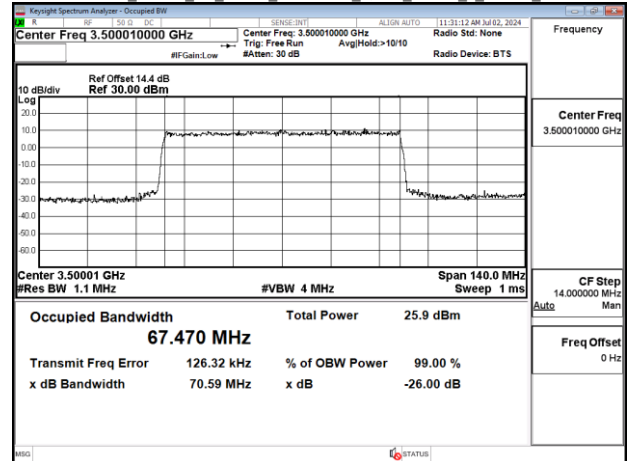
Band77-Part27_70MHz_CP_OFDM_SCS30kHz_QPSK_RB189_0_Chain1_CH633334
