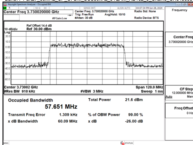
Band77-Part27 60MHz CP OFDM SCS30kHz 64QAM RB162_0 Chain0_CH656000
