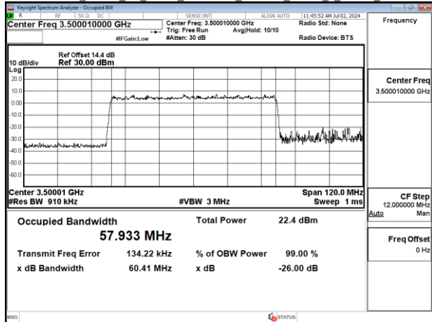
Band77-Part27 60MHz CP OFDM SCS30kHz 256QAM RB162_0 Chain1_CH633334
