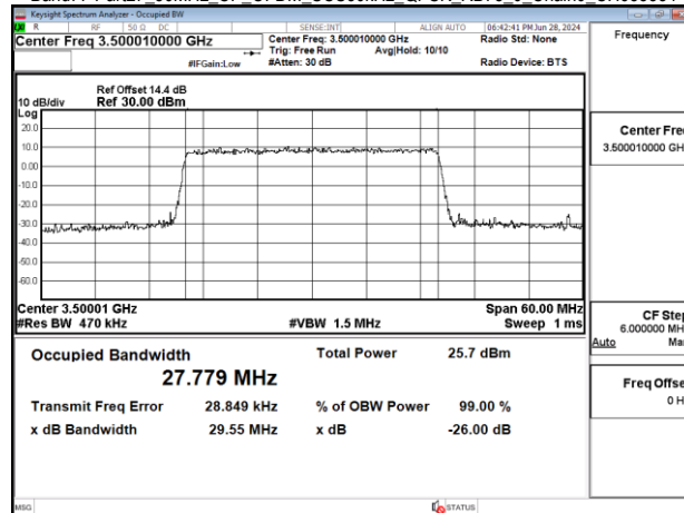
Band77-Part27_30MHz_CP_OFDM_SCS30kHz_QPSK_RB78_0_Chain0_CH633334
