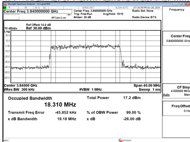
Band77-Part27_20MHz CP OFDM SCS30kHz 256QAM RB51_0 Chain0_CH656000
