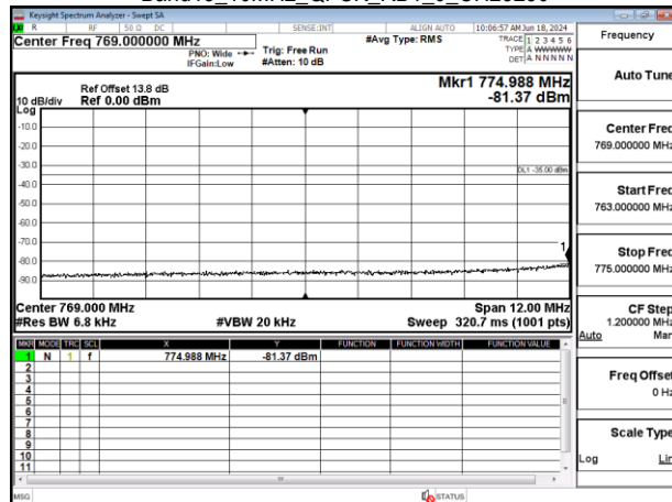
Band13_10MHz_QPSK_RB1_0_CH23230
