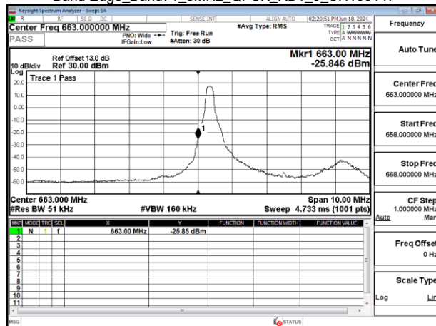
Band Edge_Band71_5MHz_QPSK_RB1_0_CH133147
