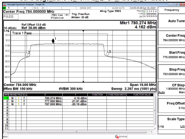
Band Edge_Band13_10MHz_QPSK_RB50_0_CH23230
