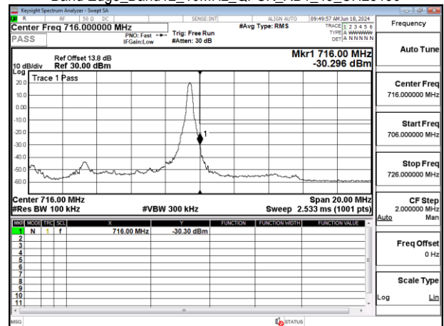
Band Edge_Band12_10MHz_QPSK_RB1_49_CH23130
