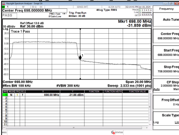
Band Edge_Band71_15MHz_QPSK_RB1_0_CH133197
