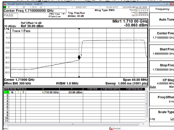
Band Edge_Band66_20MHz_QPSK_RB100_0_CH132572
