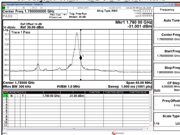
Band Edge_Band66_20MHz_QPSK_RB1_99_CH132572
