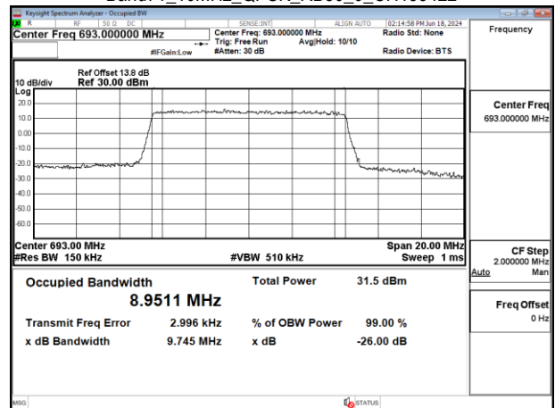
Band71_10MHz_QPSK_RB50_0_CH133422
