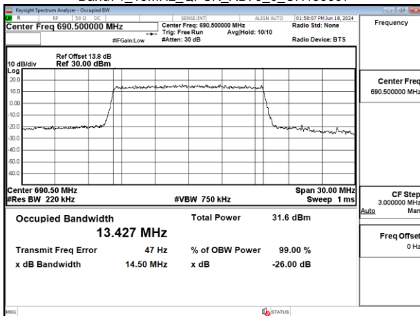
Band71_15MHz_QPSK_RB75_0_CH133397
