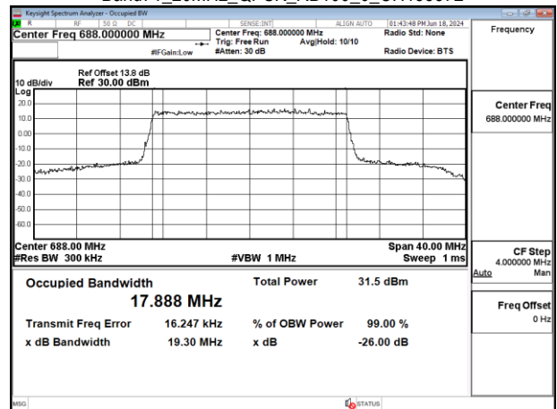
Band71_20MHz_QPSK_RB100_0_CH133372
