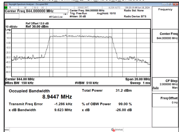
Band5_10MHz_QPSK_RB50_0_CH20600
