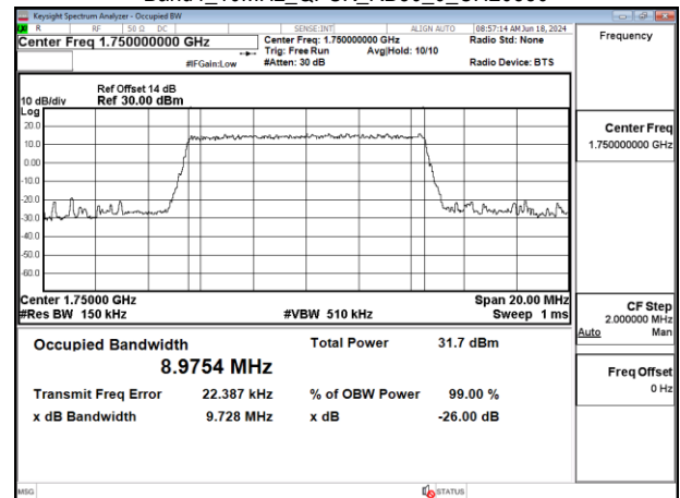
Band4_10MHz_QPSK_RB50_0_CH20350
