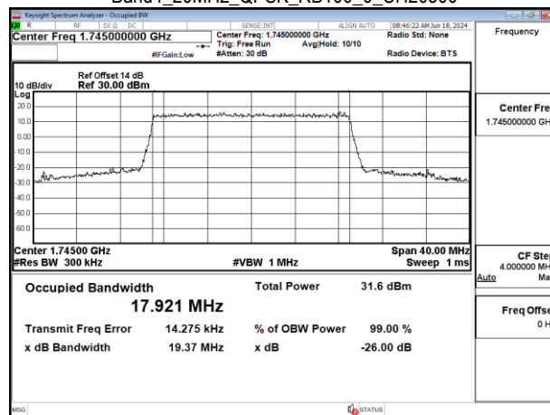
Band4_20MHz_QPSK_RB100_0_CH20300
