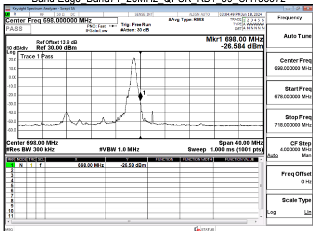
Band Edge_Band71_20MHz_QPSK_RB100_0_CH133222
