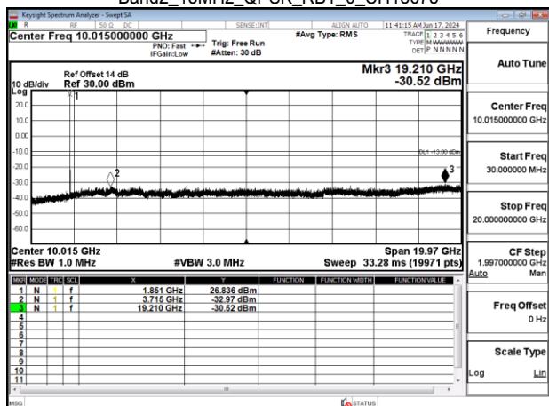
Band2_15MHz_QPSK_RB1_0_CH18900
