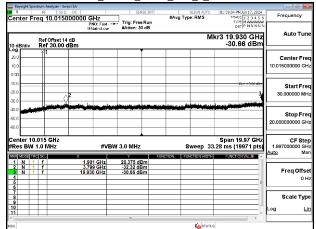
Band2_10MHz_QPSK_RB1_0_CH19150
