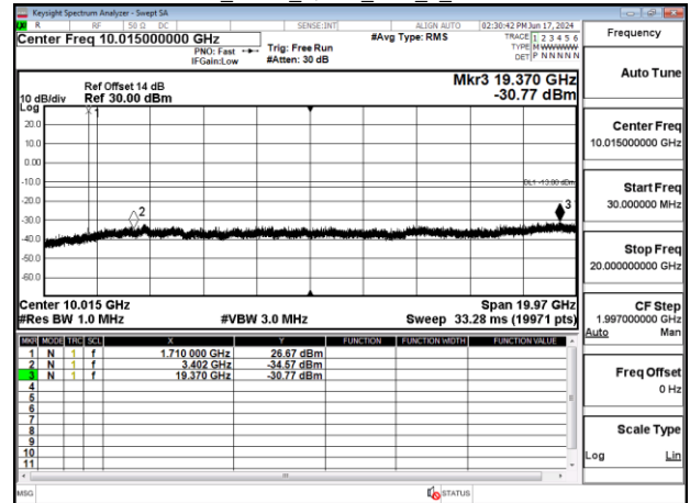
Band4_3MHz_QPSK_RB1_0_CH20175
