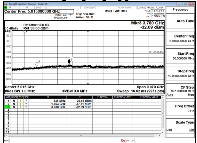
Band5_3MHz_QPSK_RB1_0_CH20635
