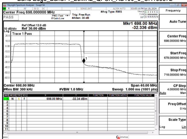
Band Edge_Band71_20MHz_QPSK_RB100_0_CH133372
