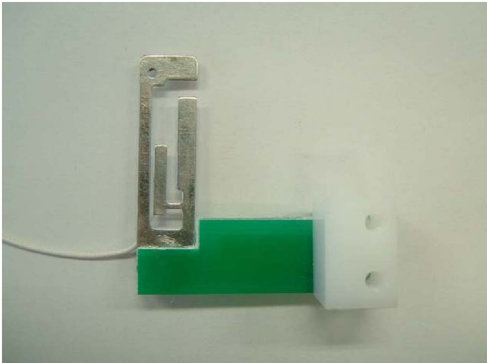
CAN4313359-REAR(Antenna)
