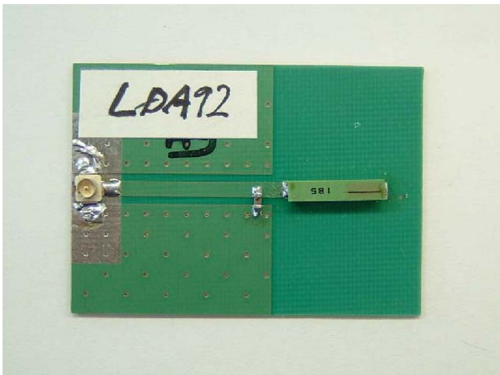
LDA92-FRONT(Antenna)
