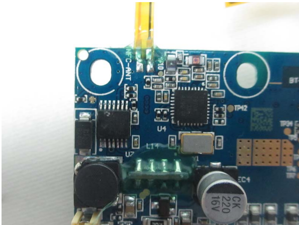
NFC module board
