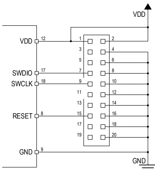
A) 20 Pin ARM Header
