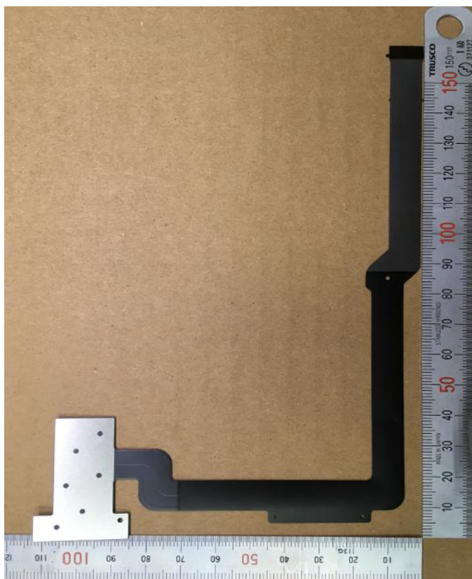
FPC_JOINT_LCD_B
