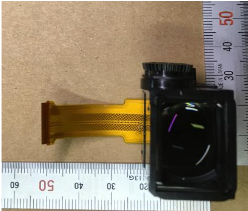
EVF_A
