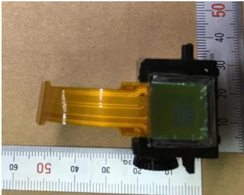
EVF_B
