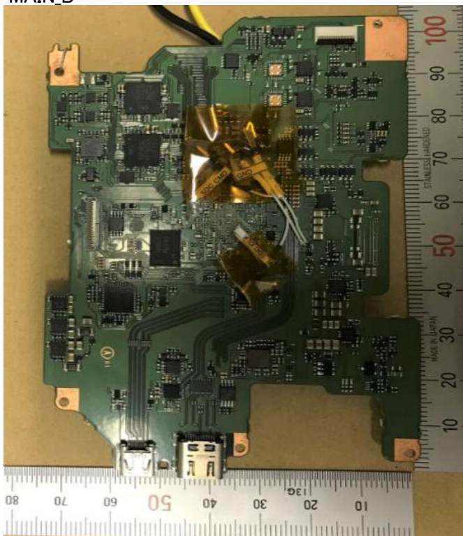
MAIN_B
