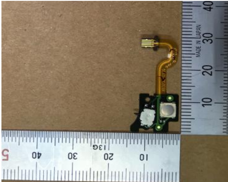
FPC_AF_A
