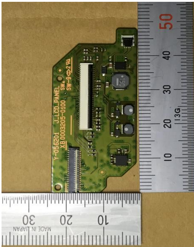
FPC_JOINT_LCD_A
