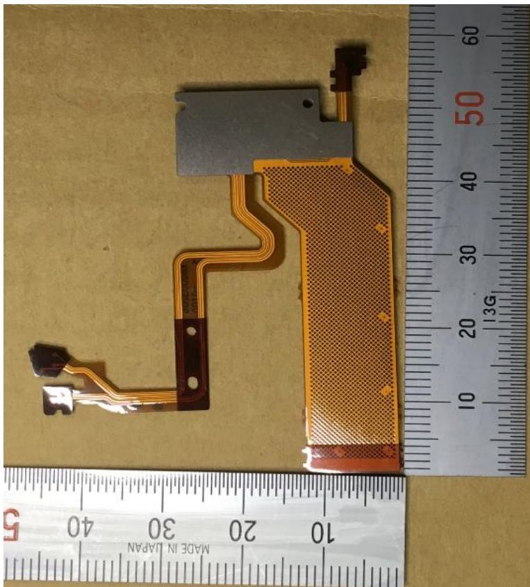
FPC_JOINT_LCD_BODY_B
