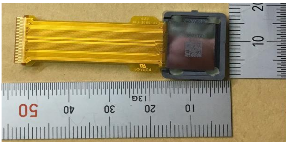
FPC_EVF_B
