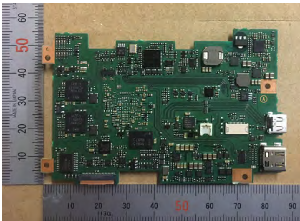
PWB MAIN_B
