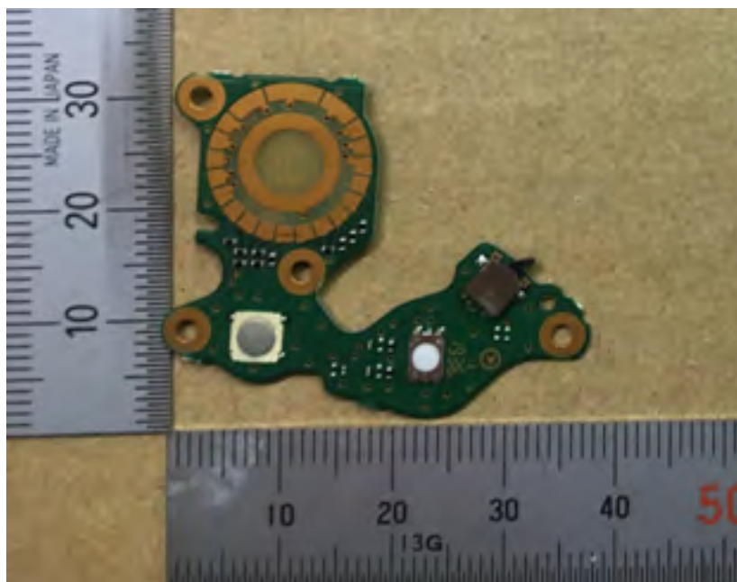
PWB TOP R_A
