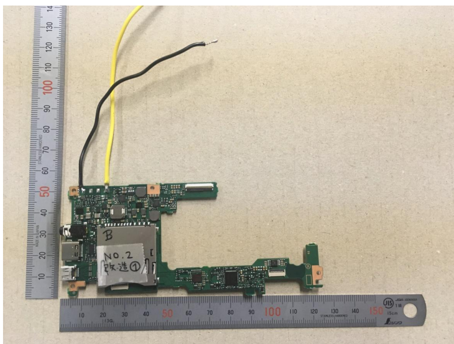
PWB_MAIN_B
