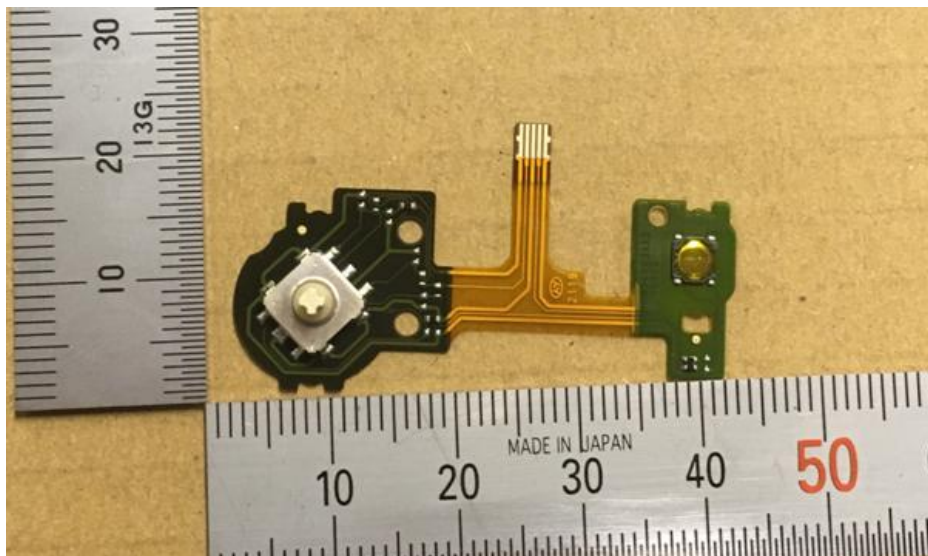
FPC_REAR_A
