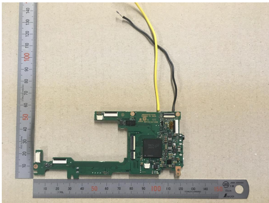
PWB_MAIN_B
