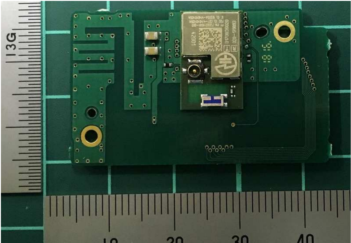
Wlan Module PCB
