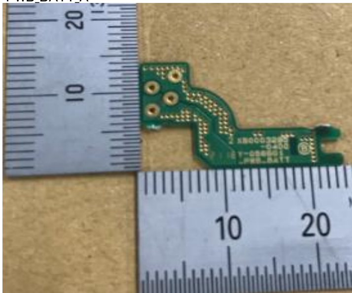
PWB_BATT_A
