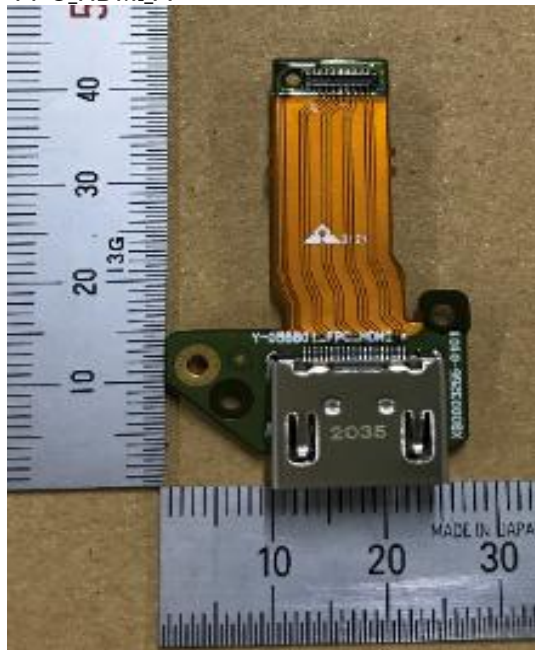
FPC.HDMI.A
