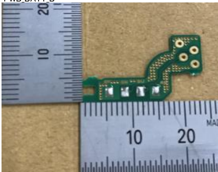
PWB_BATT_B
