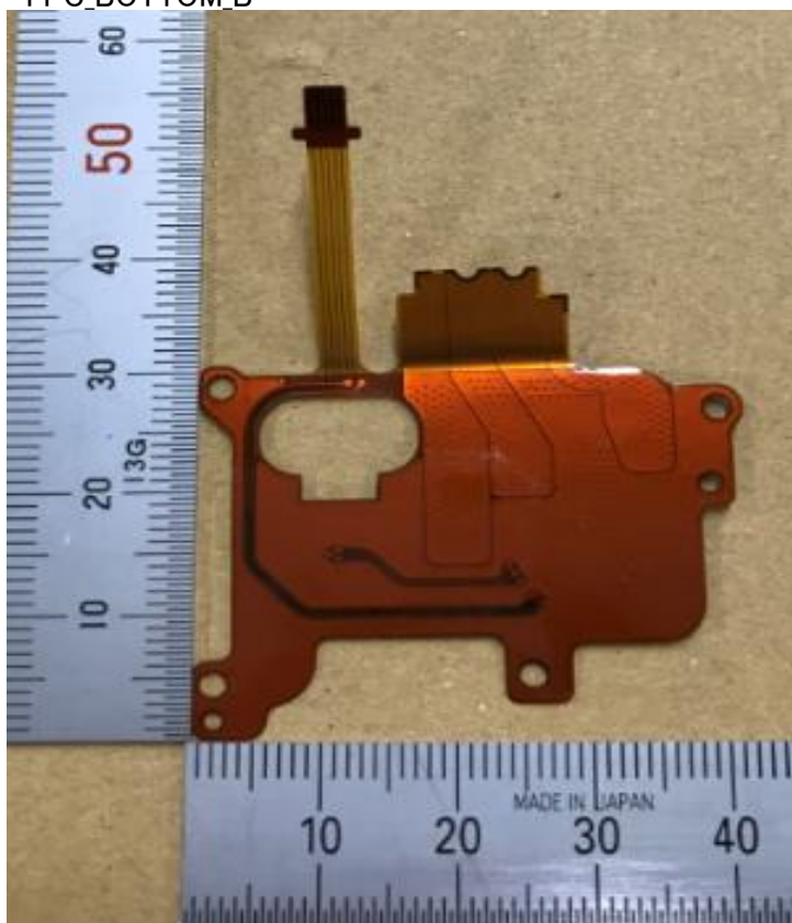
FPC_BOTTOM_B
