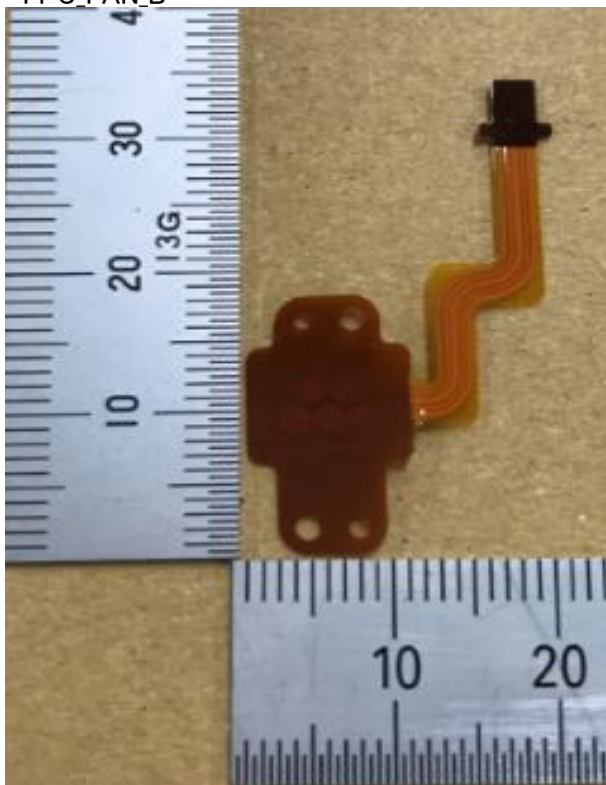
FPC_FAN_B
