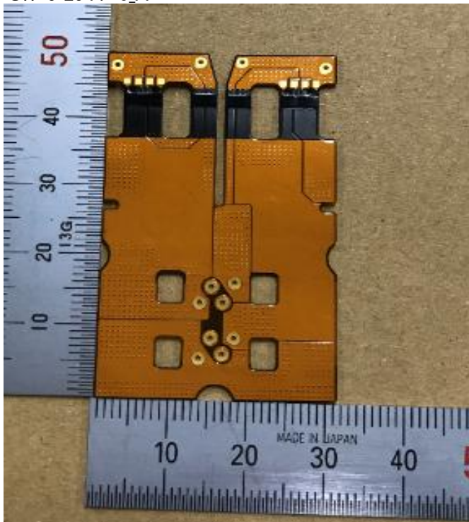
SW-9 294V-0.A
