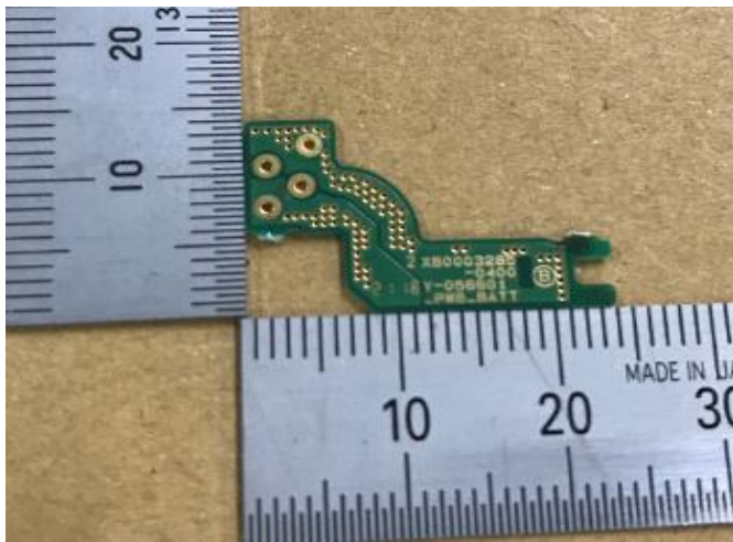
PWB_BATT_A
