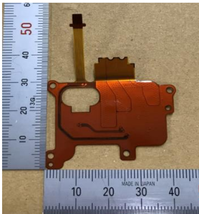
FPC_BOTTOM_B
