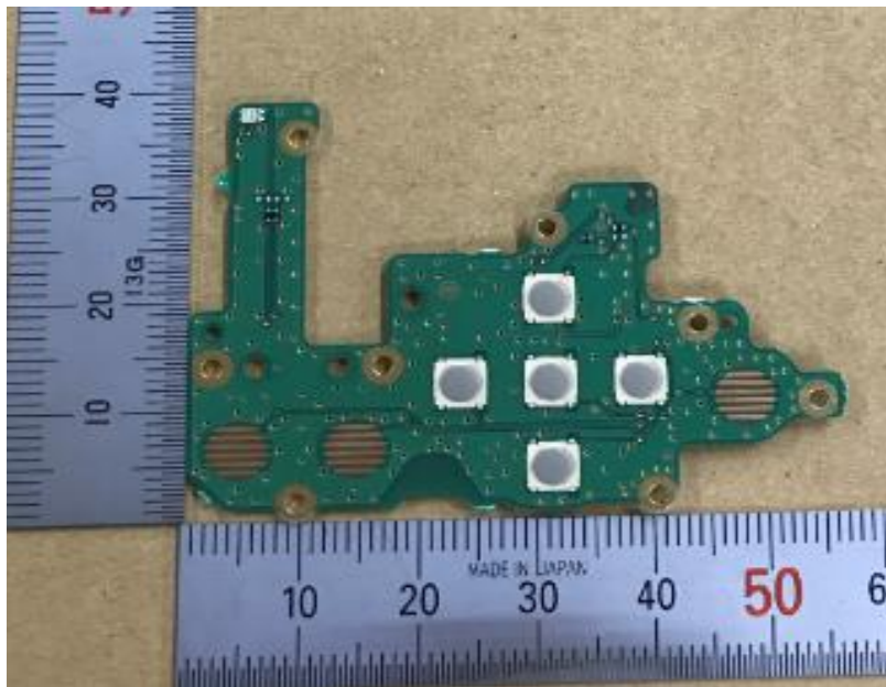
PWB_REAR_A
