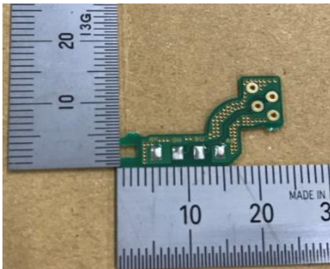
PWB_BATT_B
