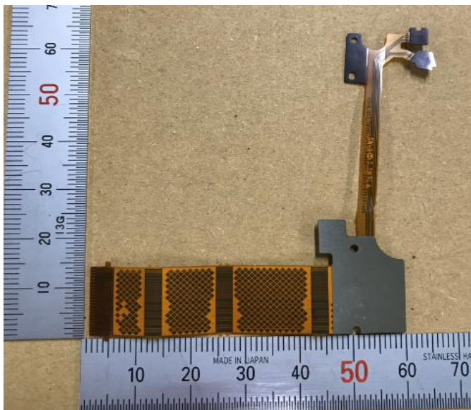
FPC_JOINT_LCD_BODY_B
