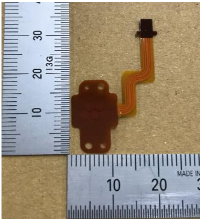
FPC_FAN_B
