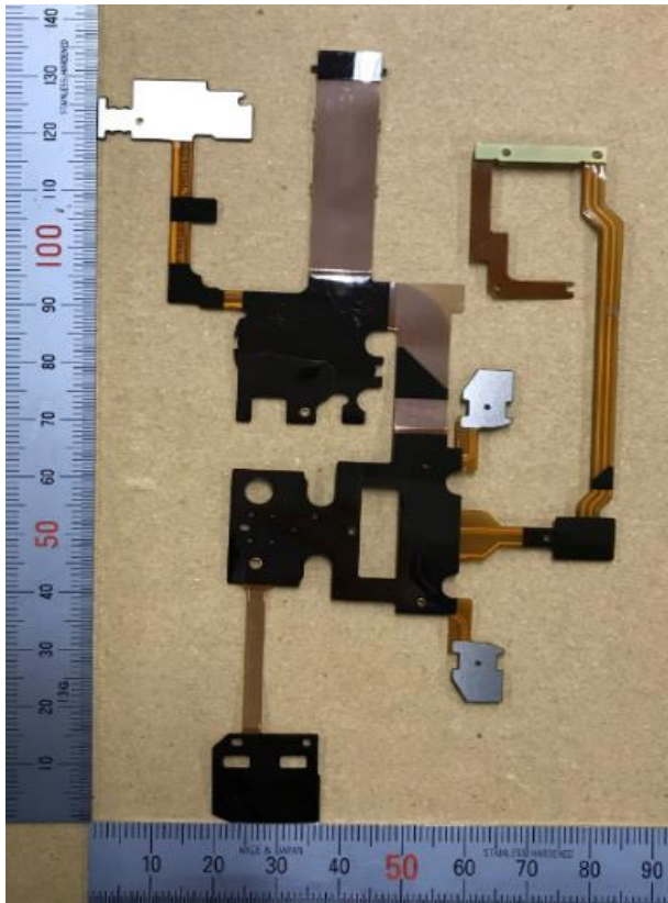
FPC_TOP_LB
