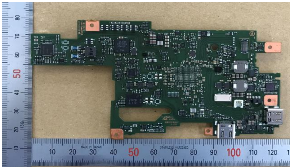
MAIN_B
