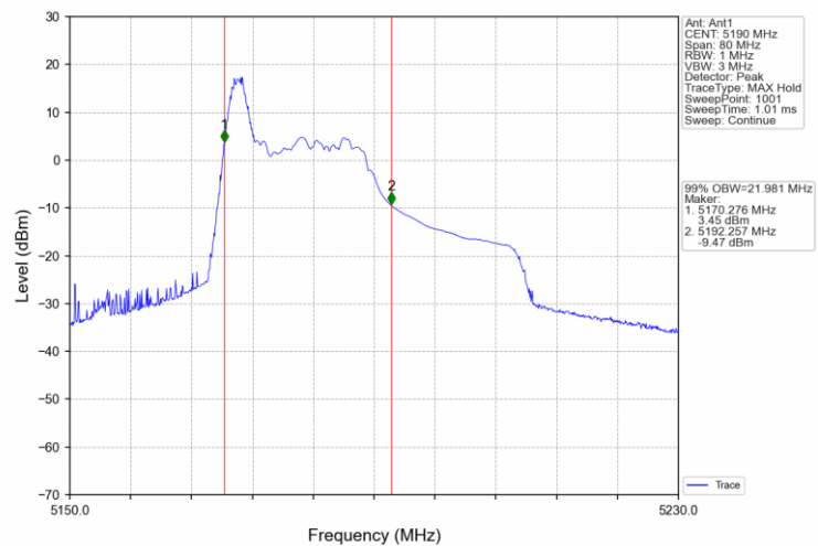
802.11ax(HEW40) LCH 5190MHz RU52 37 Ant1 NTNv
