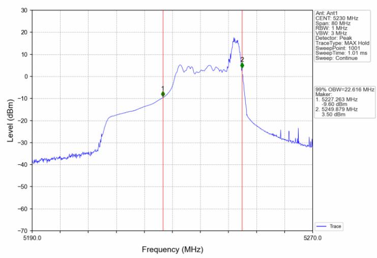
802.11ax(HEW40) HCH 5230MHz RU52 44 Ant1 NTNv
