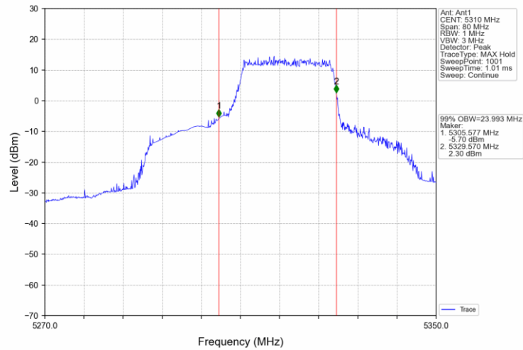
802.11ax(HEW40)_HCH_5310MHz_RU484_65_Ant1_NTNV
