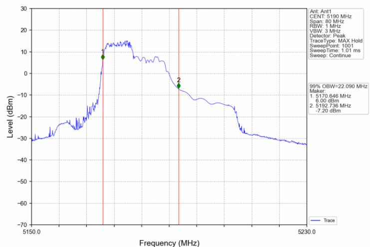
802.11ax(HEW40) LCH 5190MHz RU242 61 Ant1 NTNv
