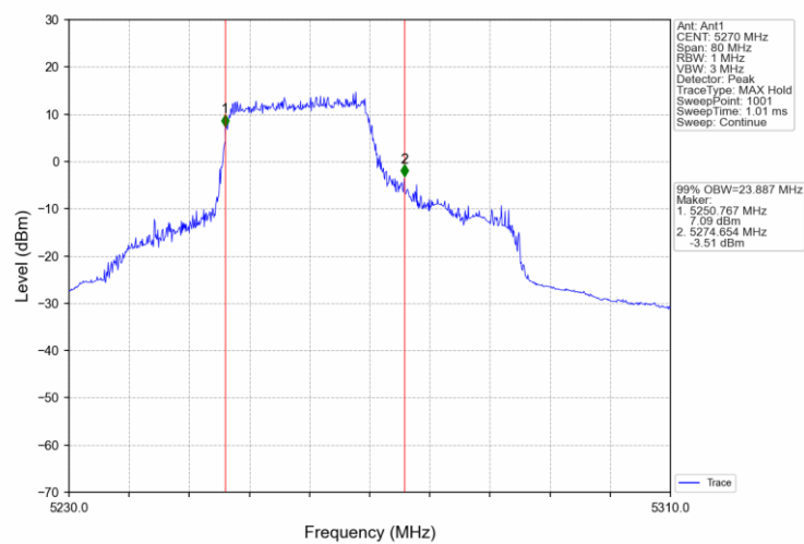
802.11ax(HEW40) LCH 5270MHz RU484 65 Ant1 NTNv
