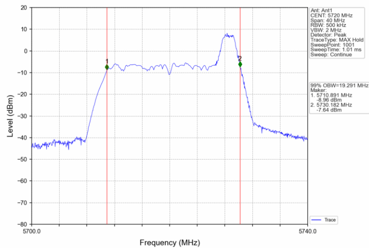
802.11ax(HEW20)_HCH_5720MHz_RU52_40_Ant1_NTNV
