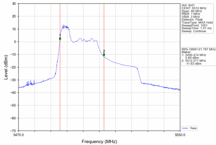
802.11ax(HEW40) LCH 5510MHz RU106_53 Ant1 NTNv
