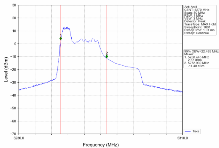
802.11ax(HEW40) LCH 5270MHz RU106_53 Ant1 NTNv
