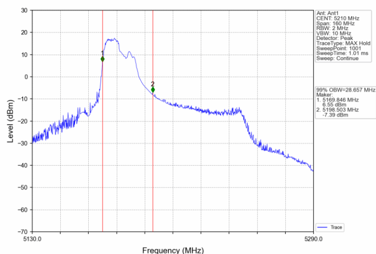
802.11ax(HEW80)_MCH_5210MHz_RU242_61_Ant1_NTNV
