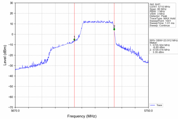
802.11ax(HEW40)_HCH_5710MHz_RU484_65_Ant1_NTNV
