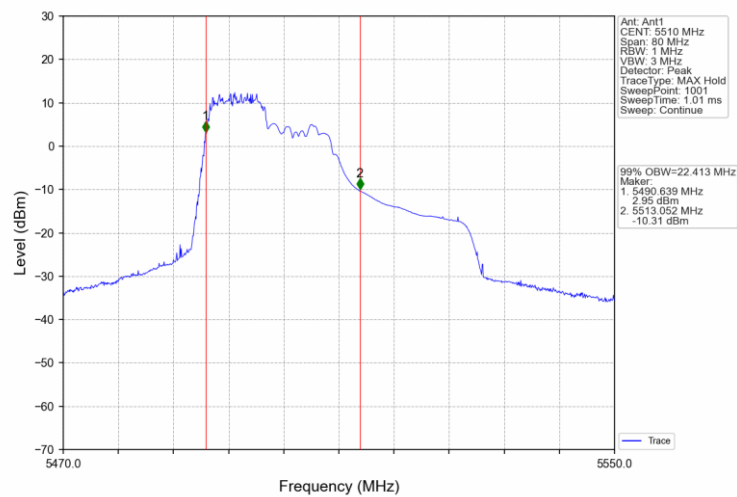
802.11ax(HEW40) LCH 5510MHz RU242_61 Ant1 NTNv
