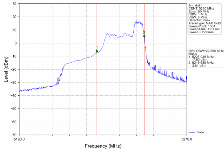
802.11ax(HEW40)_HCH_5230MHz_RU106_56_Ant1_NTNV
