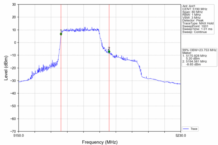
802.11ax(HEW40) LCH 5190MHz RU484 65 Ant1 NTNv
