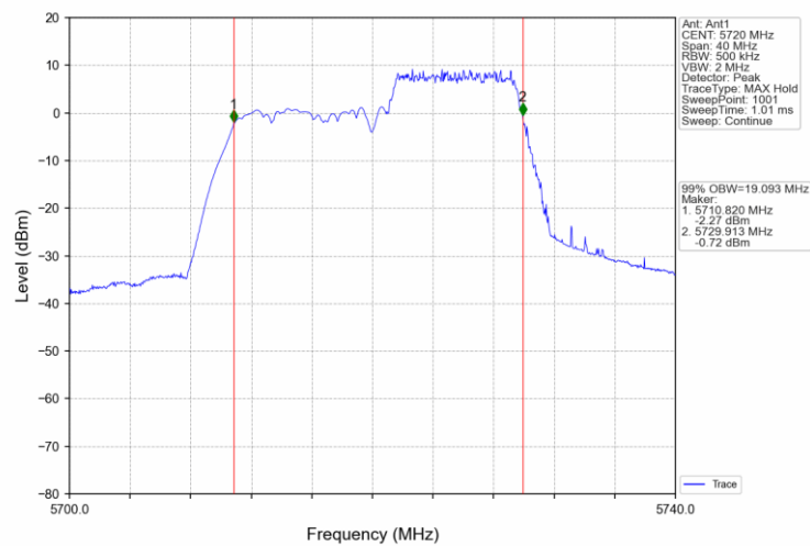
802.11ax(HEW20)_HCH_5720MHz_RU242_61_Ant1_NTNV
