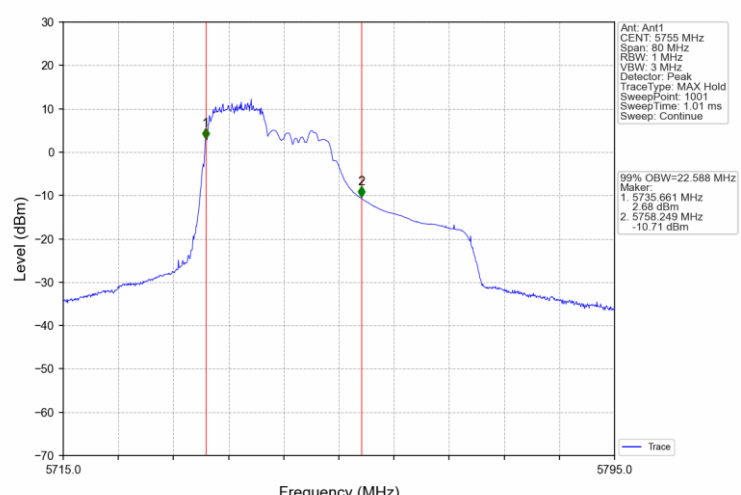
802.11ax(HEW40) LCH 5755MHz RU242 61 Ant1 NTNv
