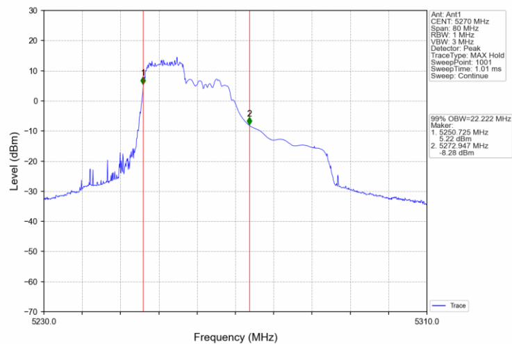
802.11ax(HEW40) LCH 5270MHz RU242 61 Ant1 NTNv
