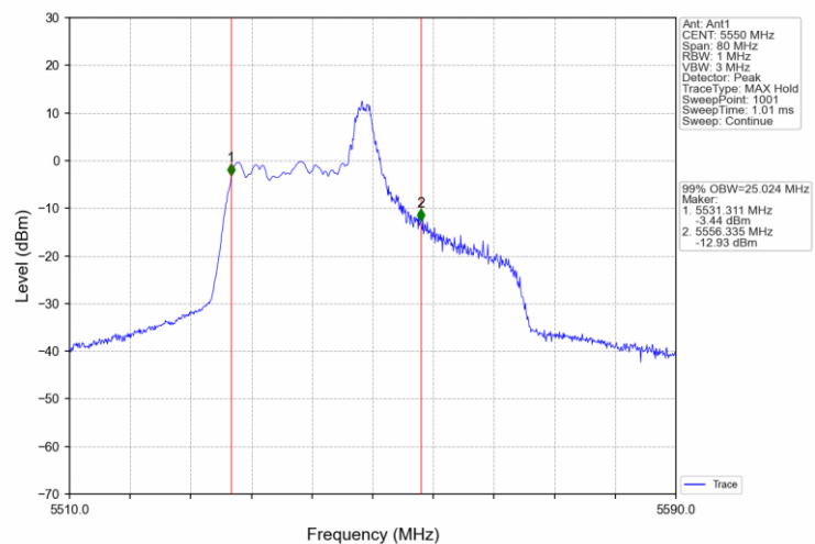
802.11ax(HEW40) MCH 5550MHz RU52 40 Ant1 NTNv
