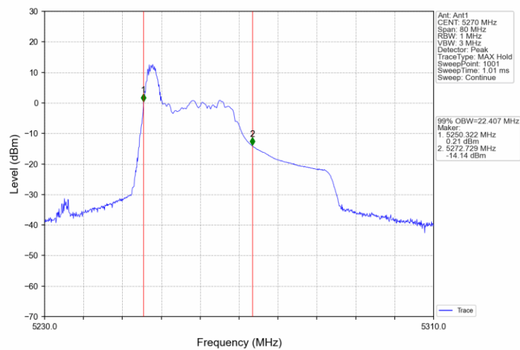
802.11ax(HEW40) LCH 5270MHz RU52_37 Ant1 NTNv
