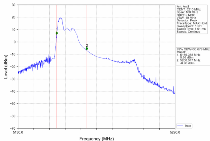
802.11ax(HEW80)_MCH_5210MHz_RU106_53_Ant1_NTNV
