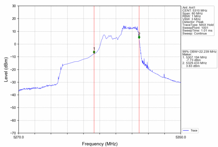
802.11ax(HEW40) HCH 5310MHz RU242_62 Ant1 NTNv
