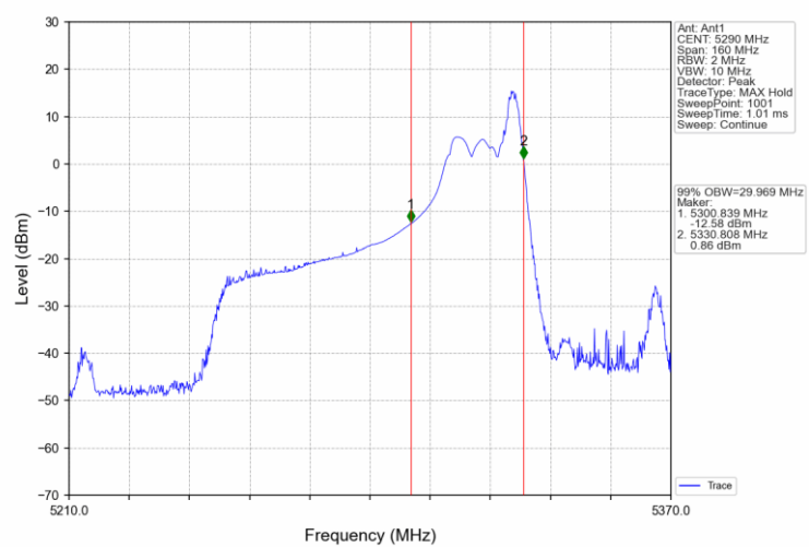
802.11ax(HEW80)_MCH_5290MHz_RU52_52_Ant1_NTNV
