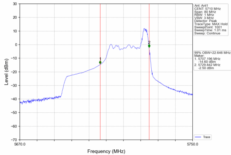
802.11ax(HEW40) HCH 5710MHz RU52_44 Ant1 NTNv
