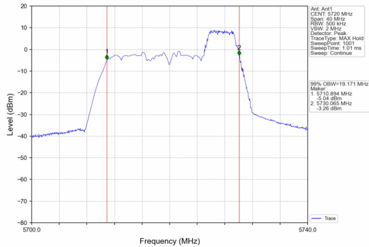
802.11ax(HEW20)_HCH_5720MHz_RU106_54_Ant1_NTNV
