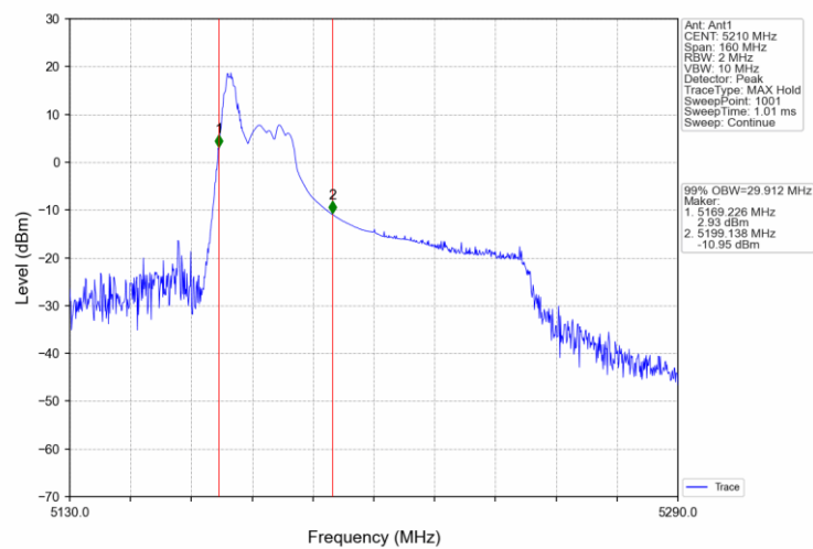
802.11ax(HEW80)_MCH_5210MHz_RU52_37_Ant1_NTNV
