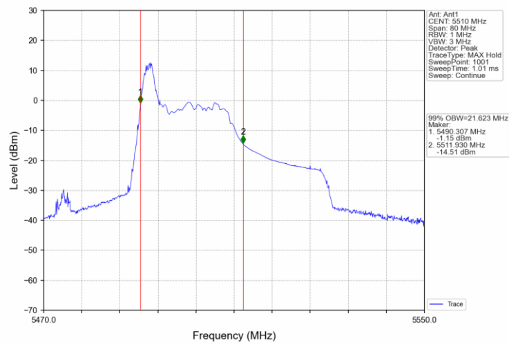
802.11ax(HEW40)_LCH_5510MHz_RU52_37_Ant1_NTNV
