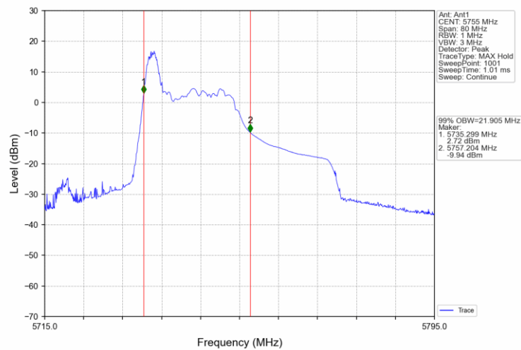
802.11ax(HEW40)_LCH_5755MHz_RU52_37_Ant1_NTNV
