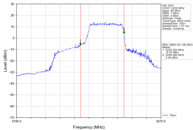
802.11ax(HEW40)_HCH_5230MHz_RU484_65_Ant1_NTNV
