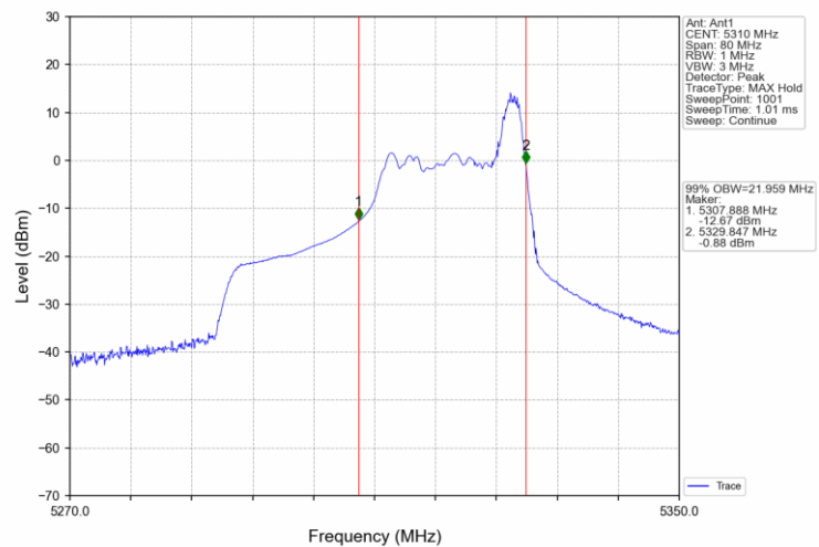
802.11ax(HEW40) HCH 5310MHz RU52_44 Ant1 NTNv
