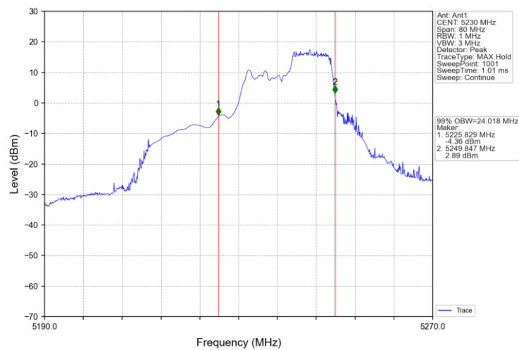
802.11ax(HEW40)_HCH_5230MHz_RU242_62_Ant1_NTNV
