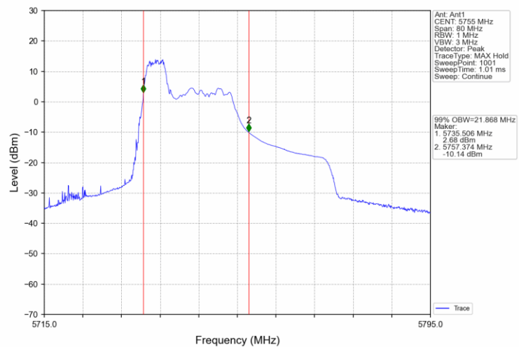
802.11ax(HEW40) LCH 5755MHz RU106 53 Ant1 NTNv
