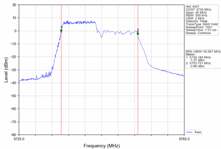
802.11ax(HEW20) LCH 5745MHz RU242_61 Ant1 NTNv
