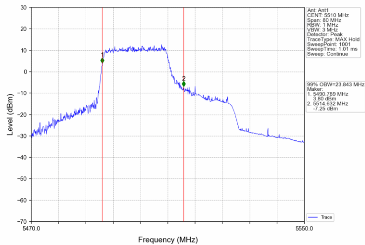
802.11ax(HEW40) LCH 5510MHz RU484_65 Ant1 NTNv
