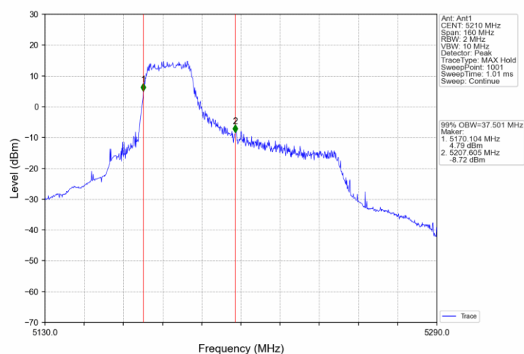
802.11ax(HEW80)_MCH_5210MHz_RU484_65_Ant1_NTNV
