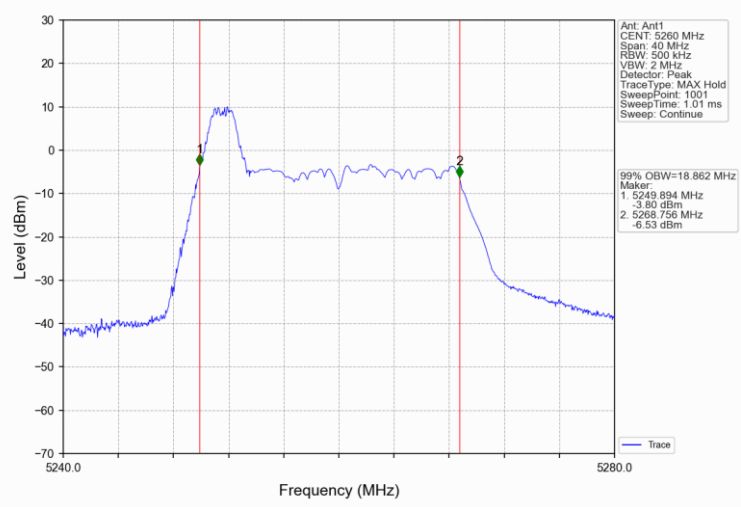
802.11ax(HEW20)_LCH_5260MHz_RU52_37_Ant1_NTNV
