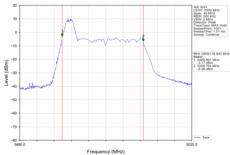
802.11ax(HEW20)_LCH_5500MHz_RU52_37_Ant1_NTNV
