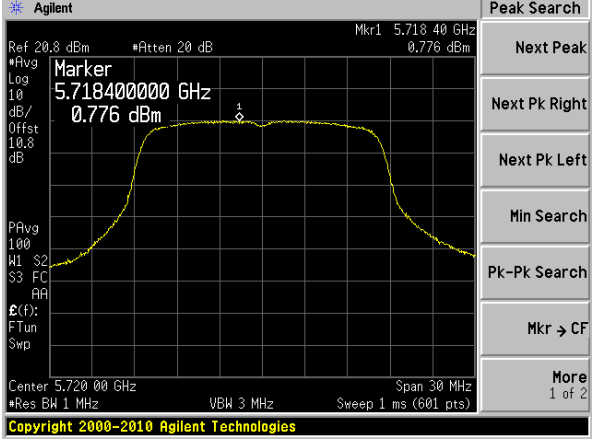
5720 MHz
