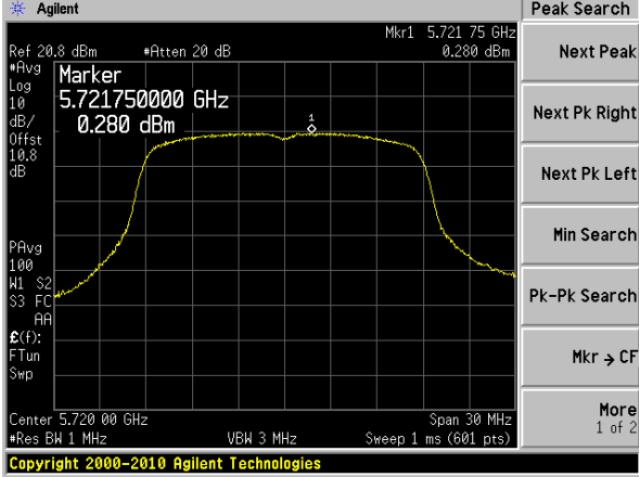
5720 MHz
