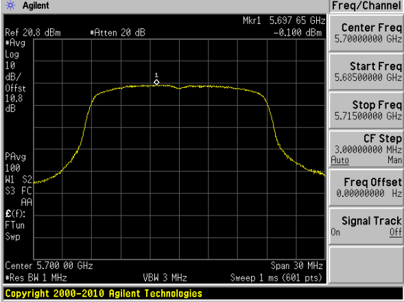
5700 MHz
