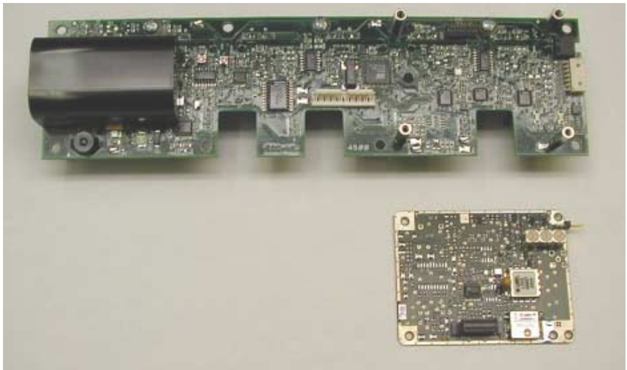
PCB Top
