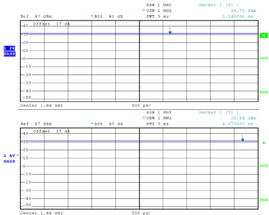
(Plot A2: GSM 1900 MHz Channel = 661)
