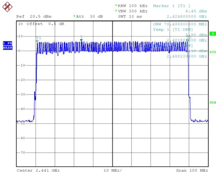
(Plot B: \pi/4 -DQPSK)
