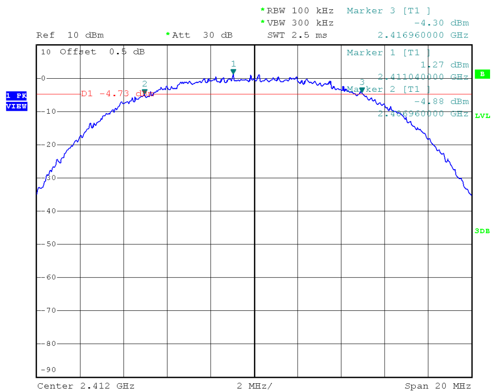
(Plot 2.3 A: Channel 1: 2412MHz @ 802.11b)
