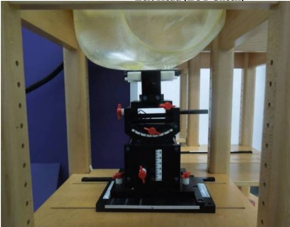
Left Head (EUT Tilt)
