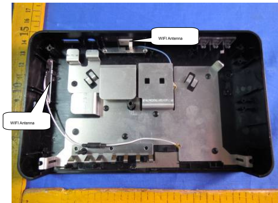
2) EUT Photo
