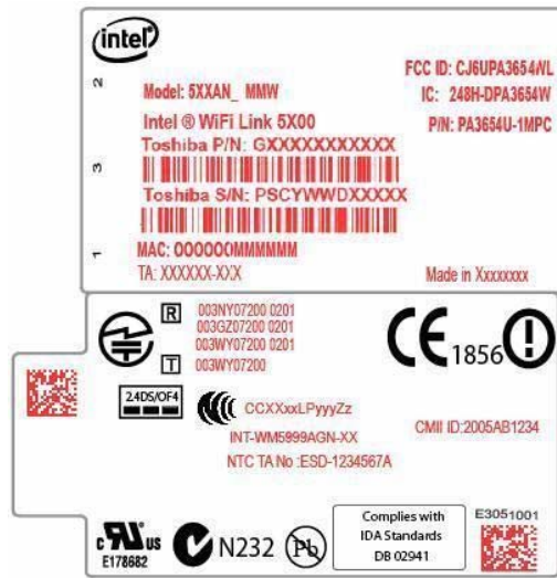
W-LAN Module label format
