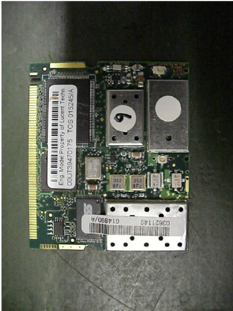
LAN modul upper side
