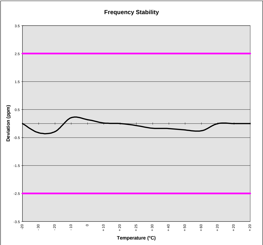
VCTCXO: VC-TCXO-204C2
