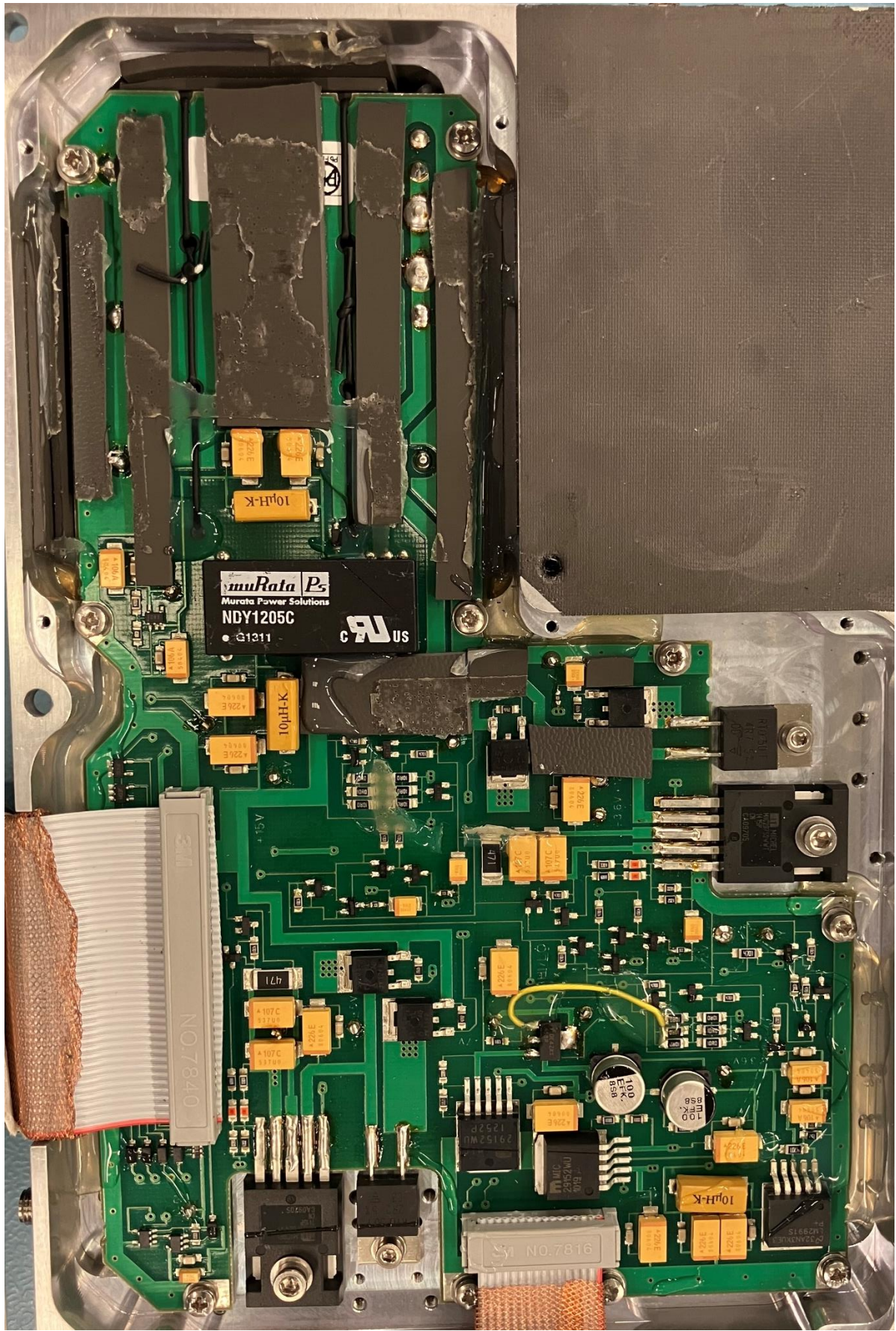
Internal – SCV HPA (PCB 001362)
