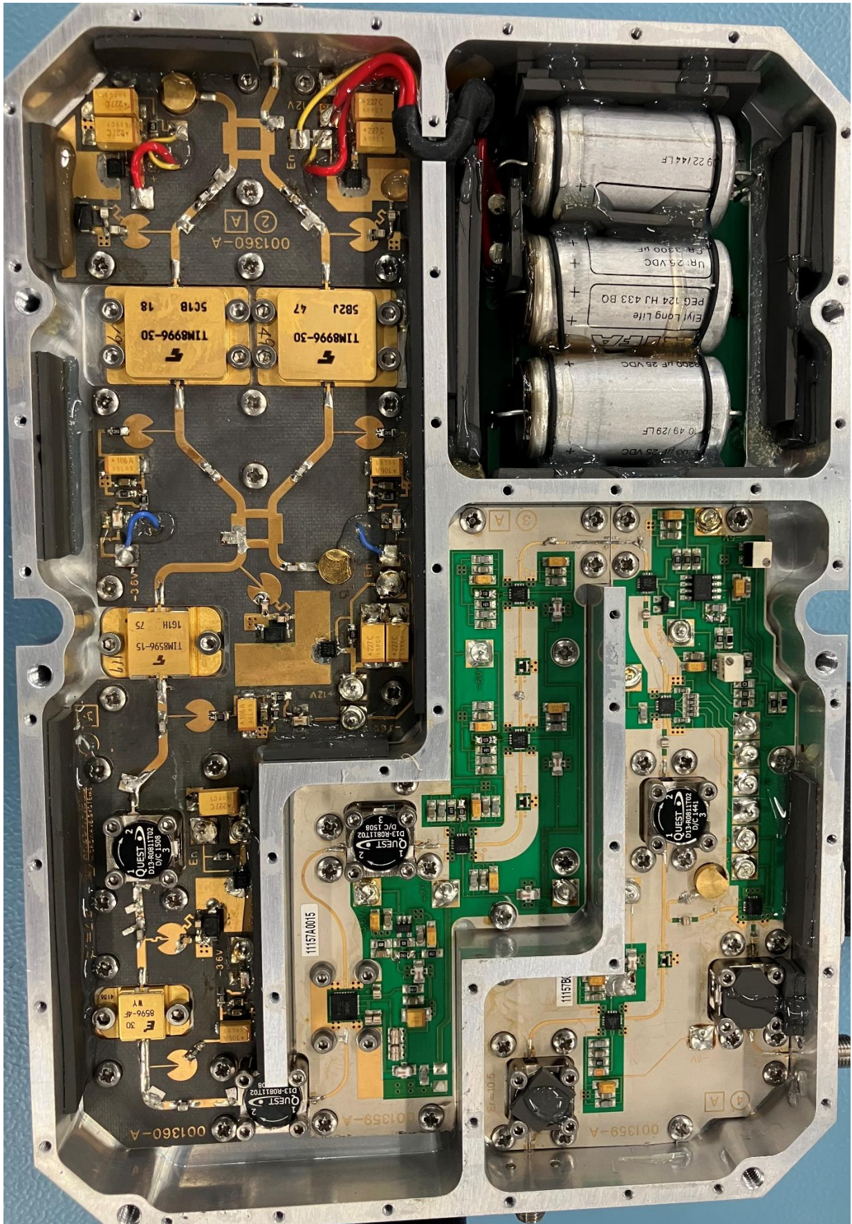
Internal – SCV HPA (PCB 001359-3, -4, 001360-1, -2, rear 001362)
