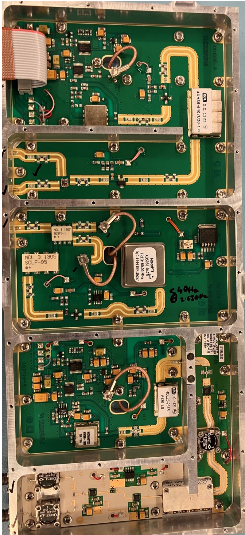
Internal – SCV Synth/PLO (PCB 001359-5, -6, -8, 001336-1, -2 )
