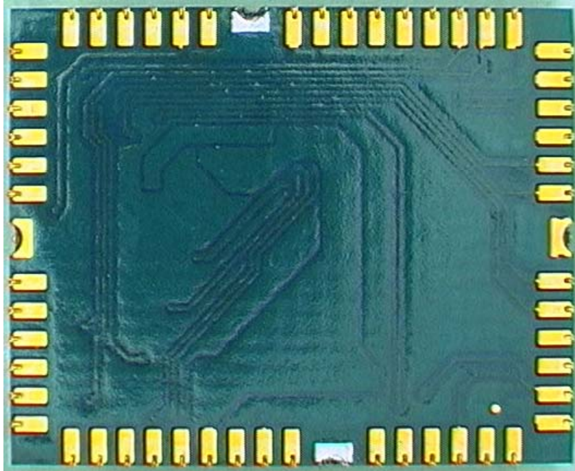
Wireless LAN Module (bottom)
