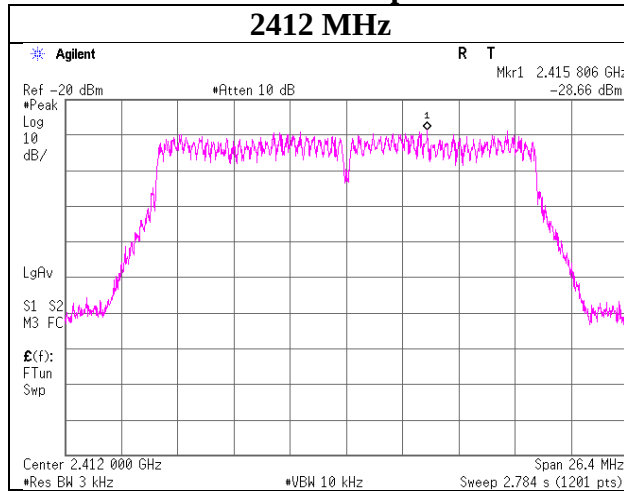
11n-20 Antenna port 1
