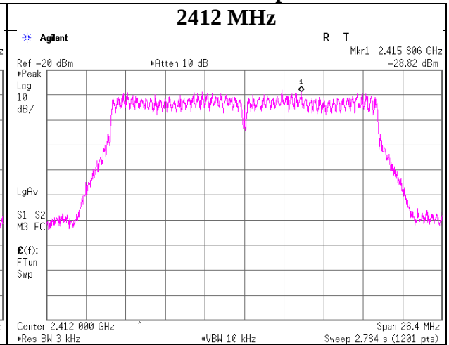
11n-20 Antenna port 2
