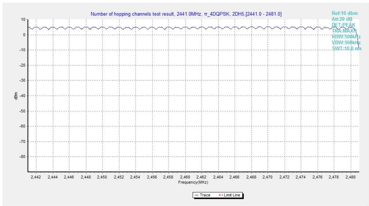
Fig. 78 Hopping channel ch40 ~ ch78 ( \pi/4 DQPSK)
