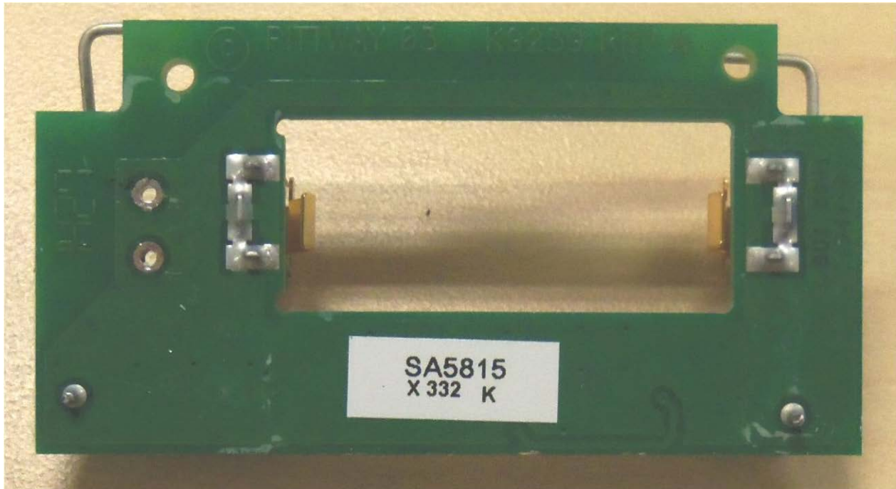
PCA BACK
